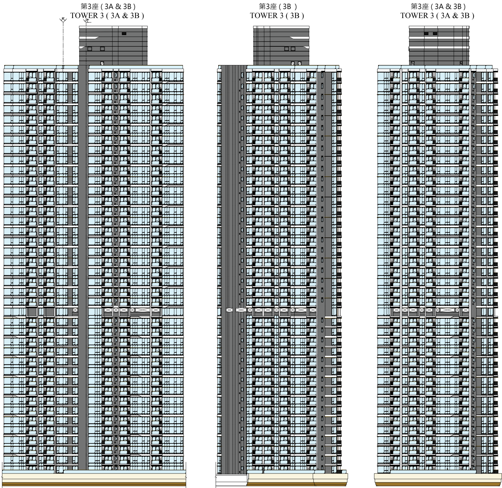
ELEVATION 1
