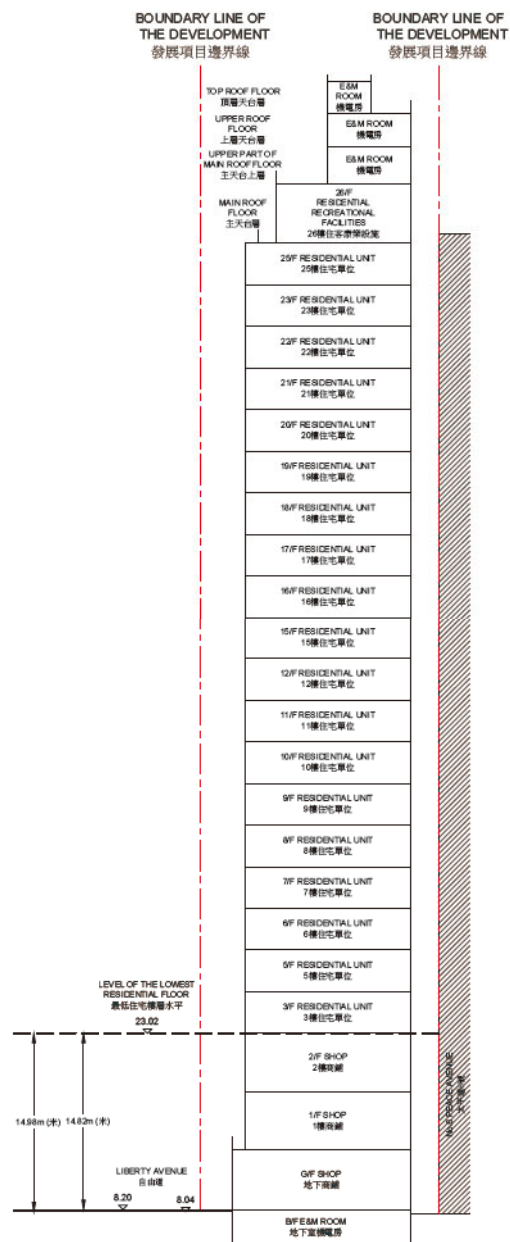
CROSS SECTION A-A 橫截面圖 A-A
