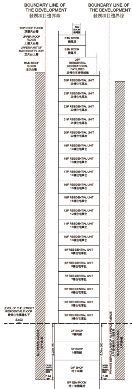
CROSS SECTION B-B 橫截面圖 B-B
