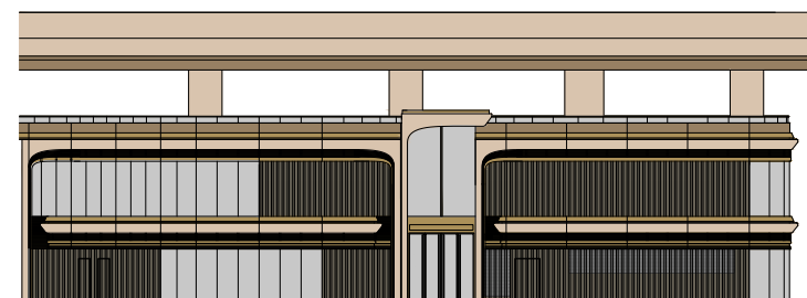
PODIUM - ELEVATION PLAN H 平台立面圖 H
