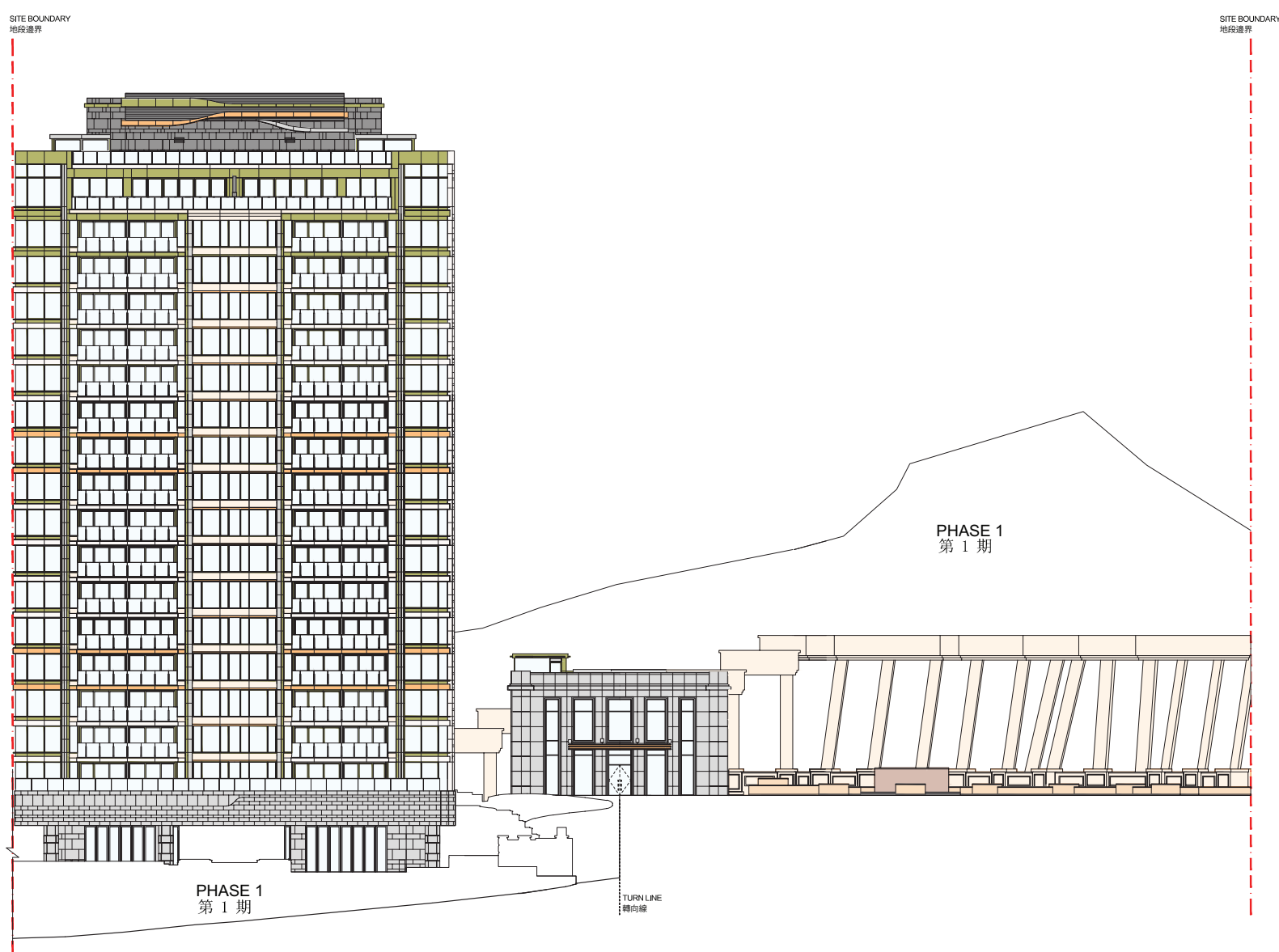
立面圖1 Elevation 1
