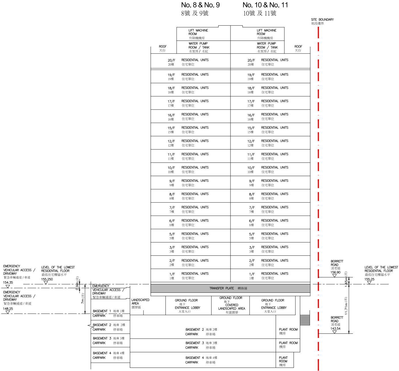
橫截面圖 C-C CROSS SECTION PLAN C-C
