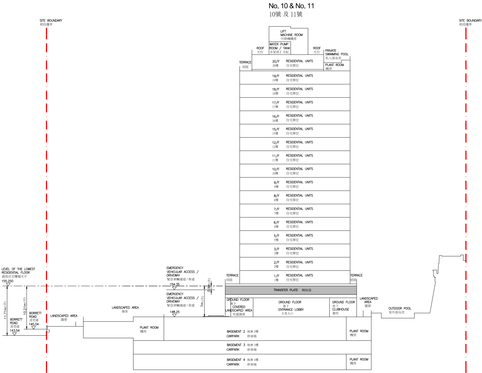
橫截面圖 B-B CROSS SECTION PLAN B-B
