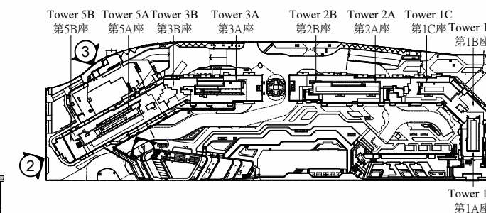
KEY PLAN 示意圖
