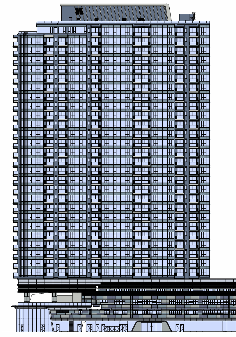
ELEVATION PLAN 1 立面圖 1
