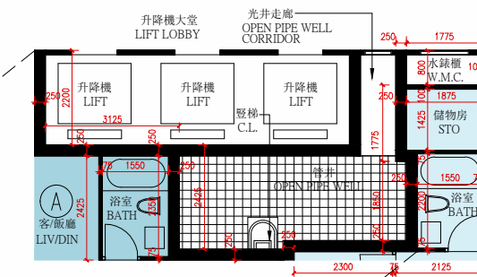
PART PLAN OF 21/F 二十一樓部分平面圖
