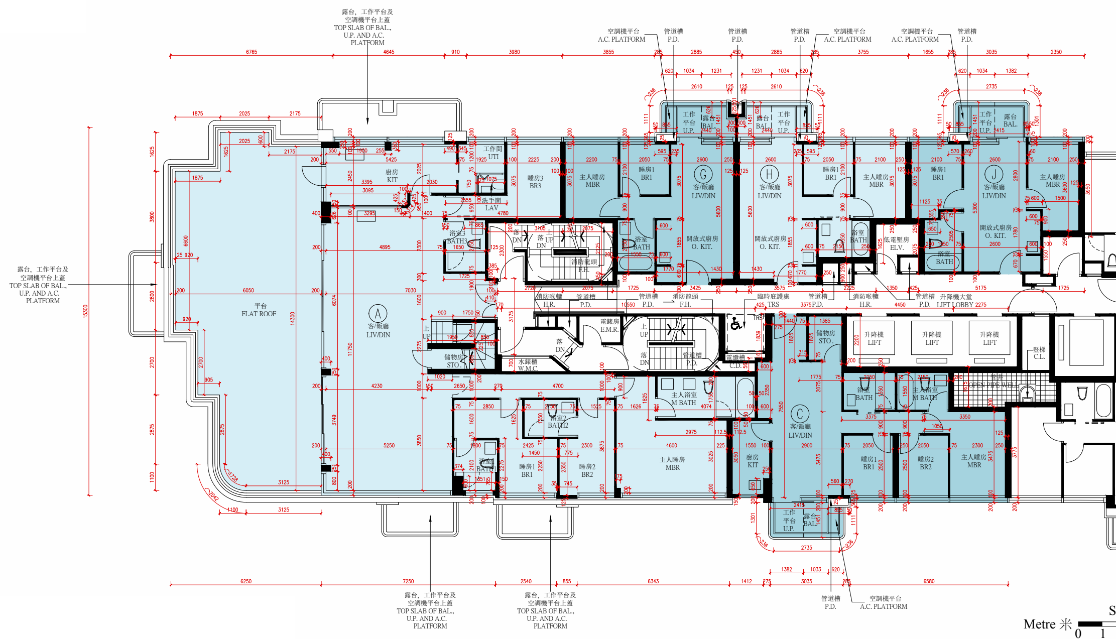
Tower 5A 第5A座
