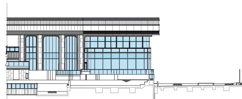
立面圖 7 Elevation Plan 7
