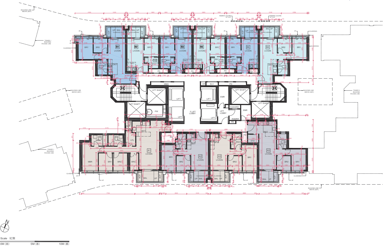
Tower 2 (Elite Zone) 28/F 第2座 (Elite Zone) 28樓
