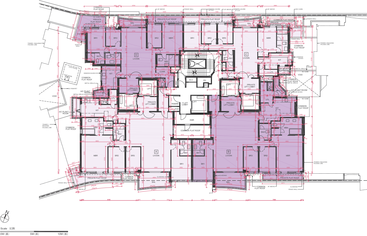
Tower 2 (Summit Tower) 32/F 第2座 (Summit Tower) 32樓
