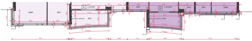
PART PLAN OF FLAT A & FLAT B ON 46/F 46樓A單位及B單位部分平面圖
