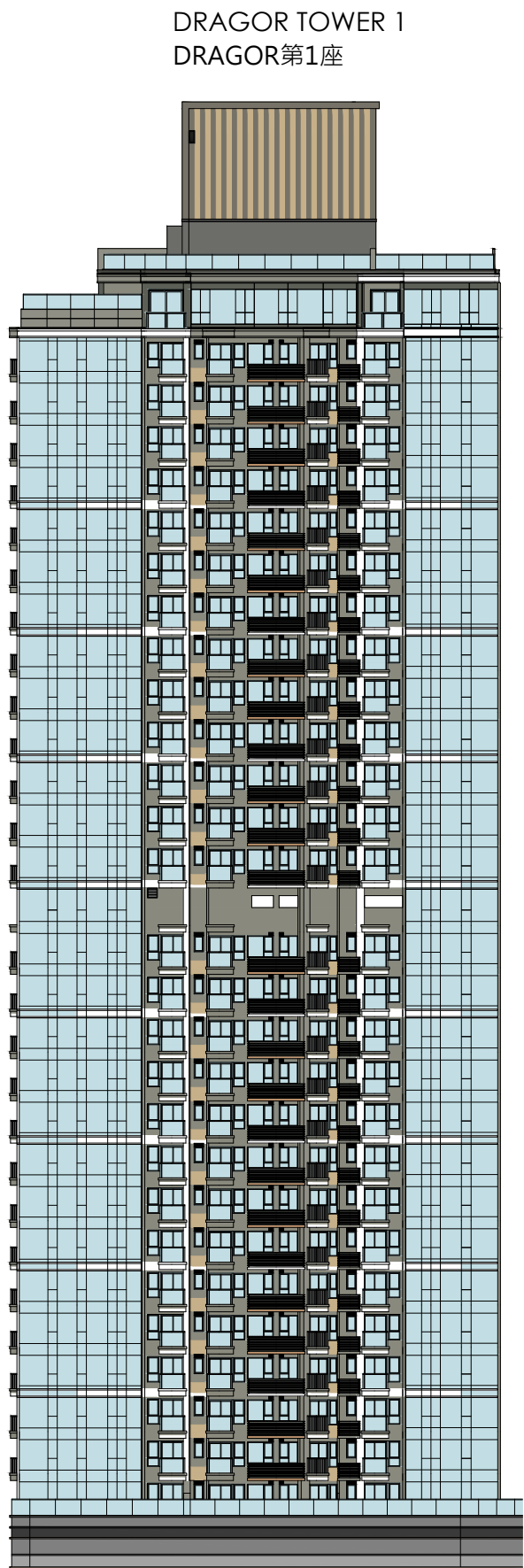
ELEVATION PLAN 1 立面圖 1
