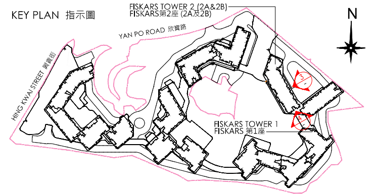
FISKARS TOWER 2 (2A&2B) FISKARS 第2座 (2A及2B)
