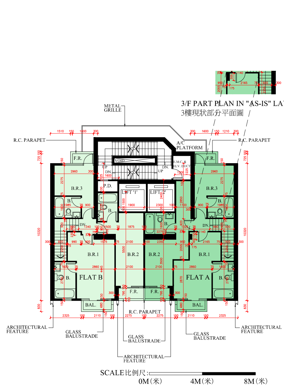
3樓平面圖 (複式高層平面圖)
