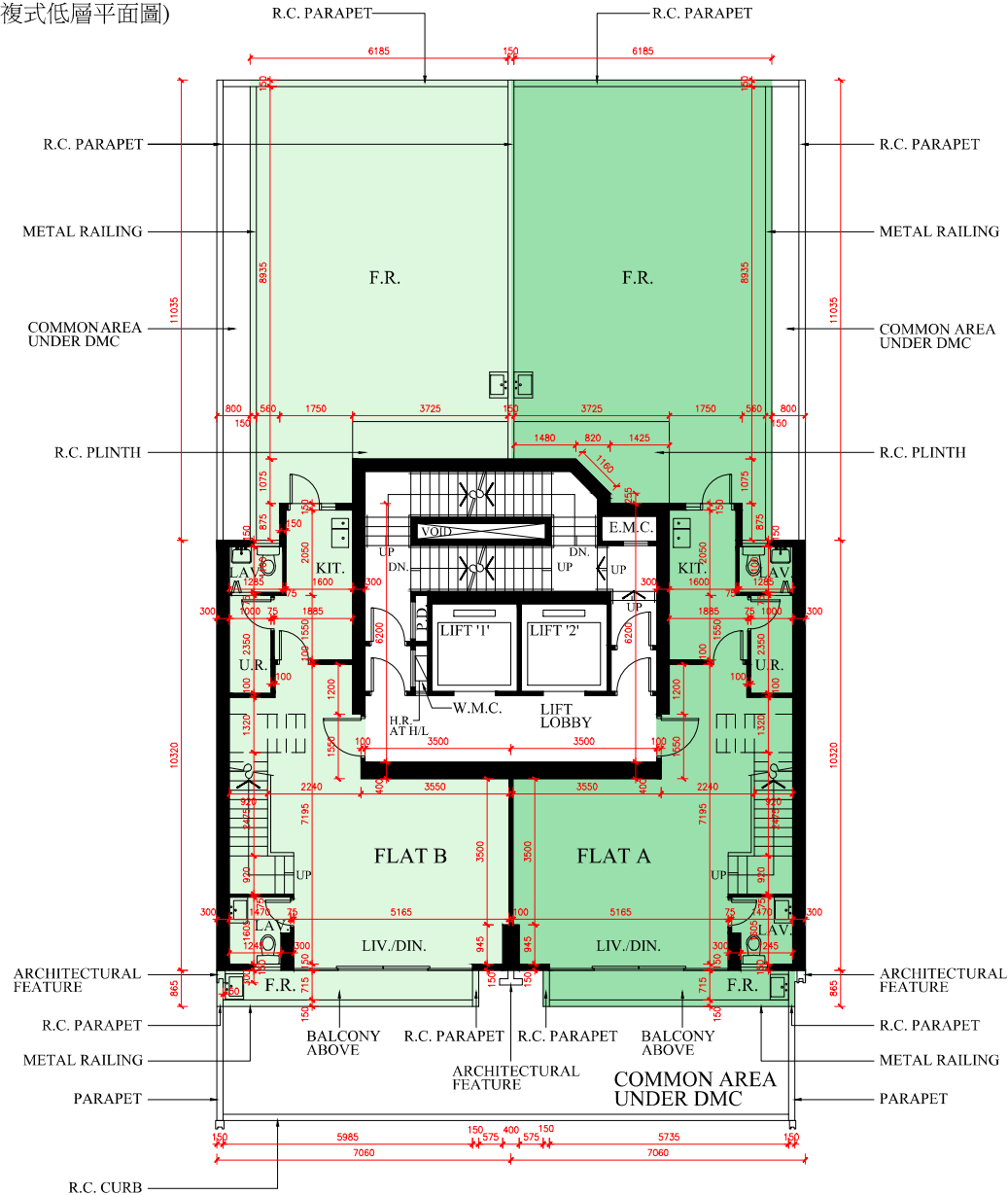
2樓平面圖 (複式低層平面圖)
