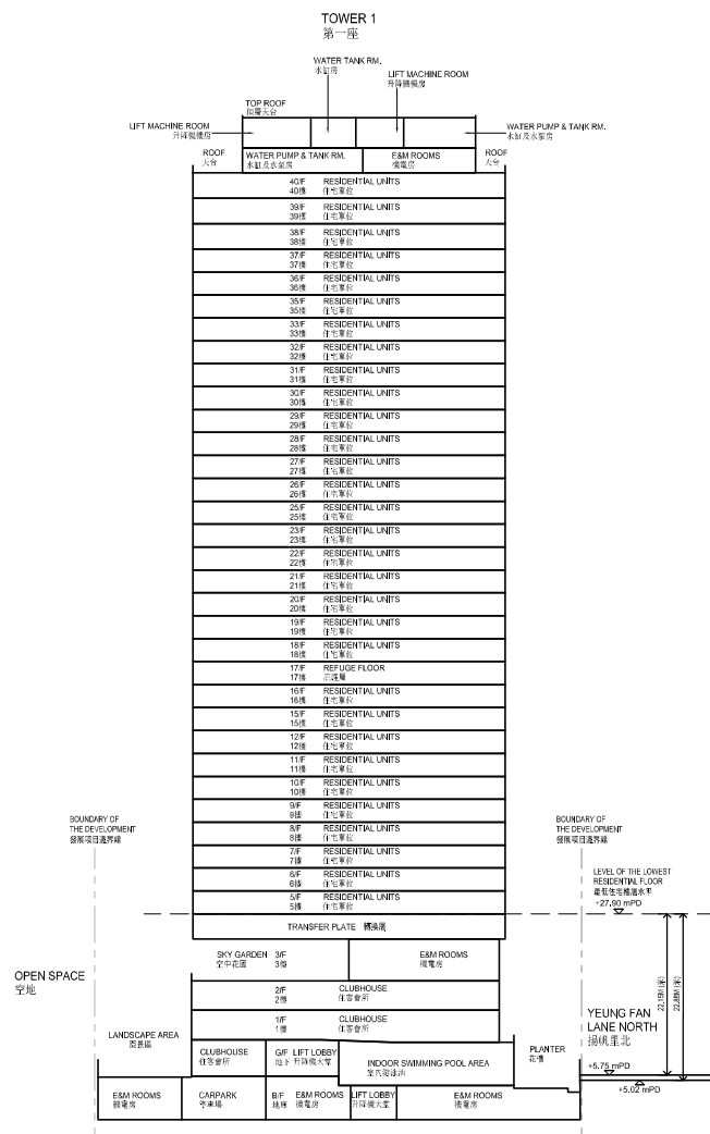
CROSS-SECTION PLAN B-B 橫截面圖 B-B
