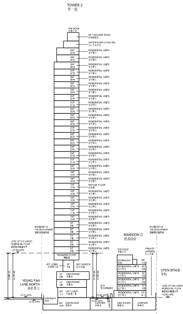
CROSS-SECTION PLAN C-C 橫截面圖 C-C
