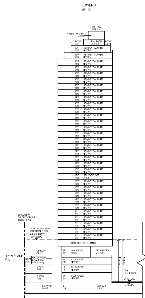
CROSS-SECTION PLAN D-D 橫截面圖 D-D
