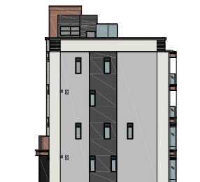
ELEVATION PLAN 2 立面圖 2
