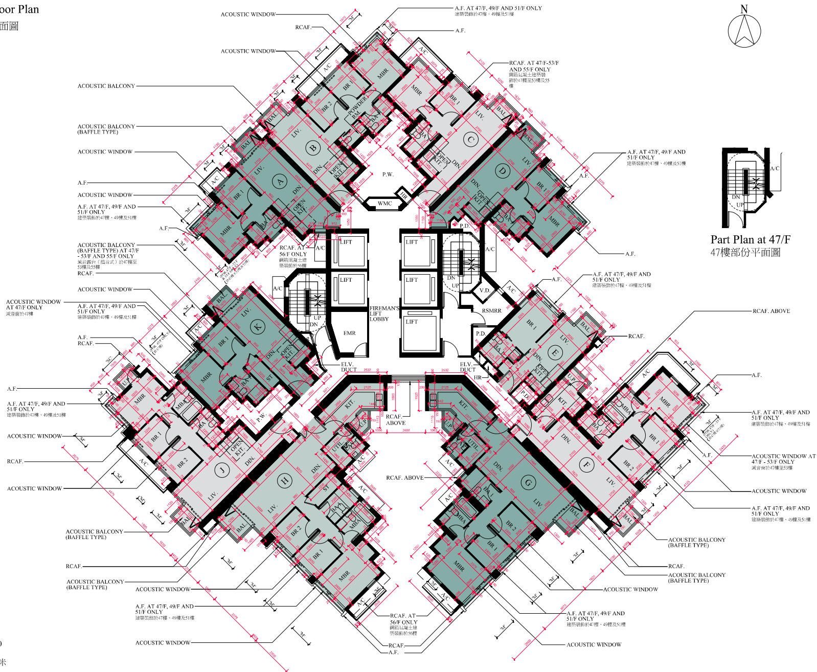
Part Plan at 47/F 47樓部份平面圖
