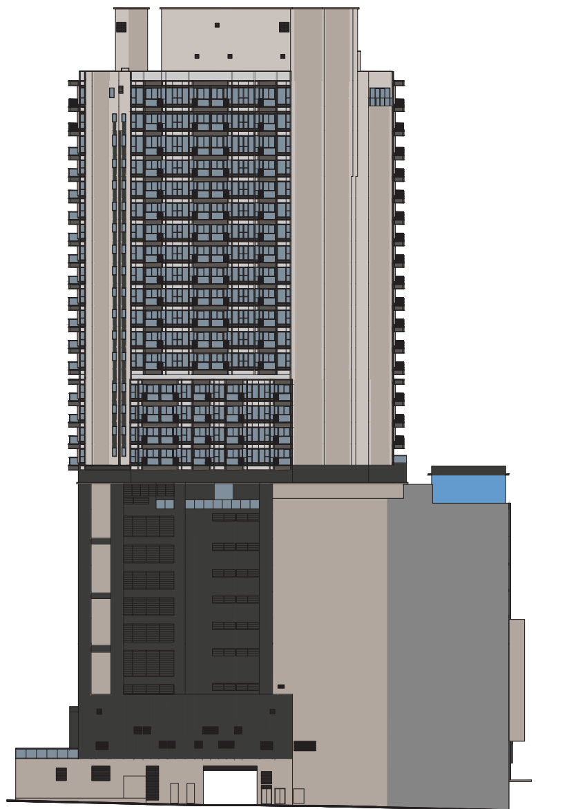
ELEVATION 3 立面 3
