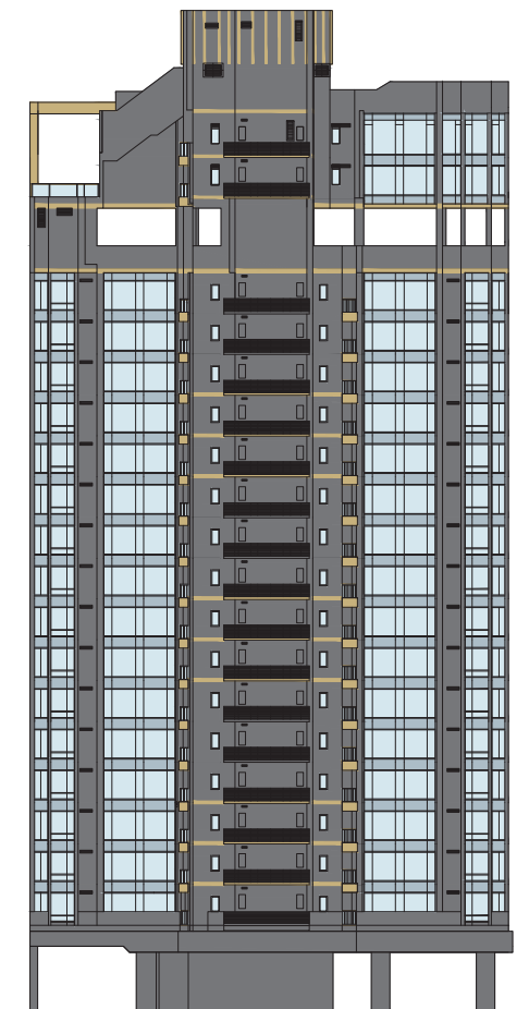
Elevation Plan 3 立面圖 3
