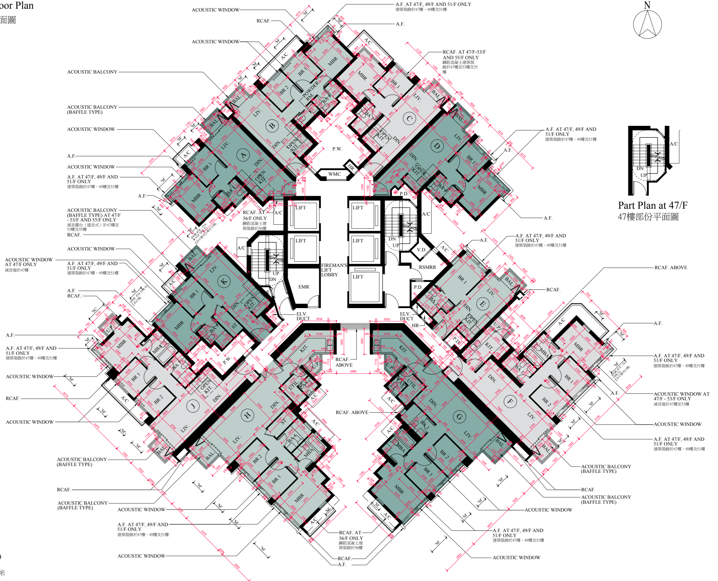
Part Plan at 47/F 47樓部份平面圖
