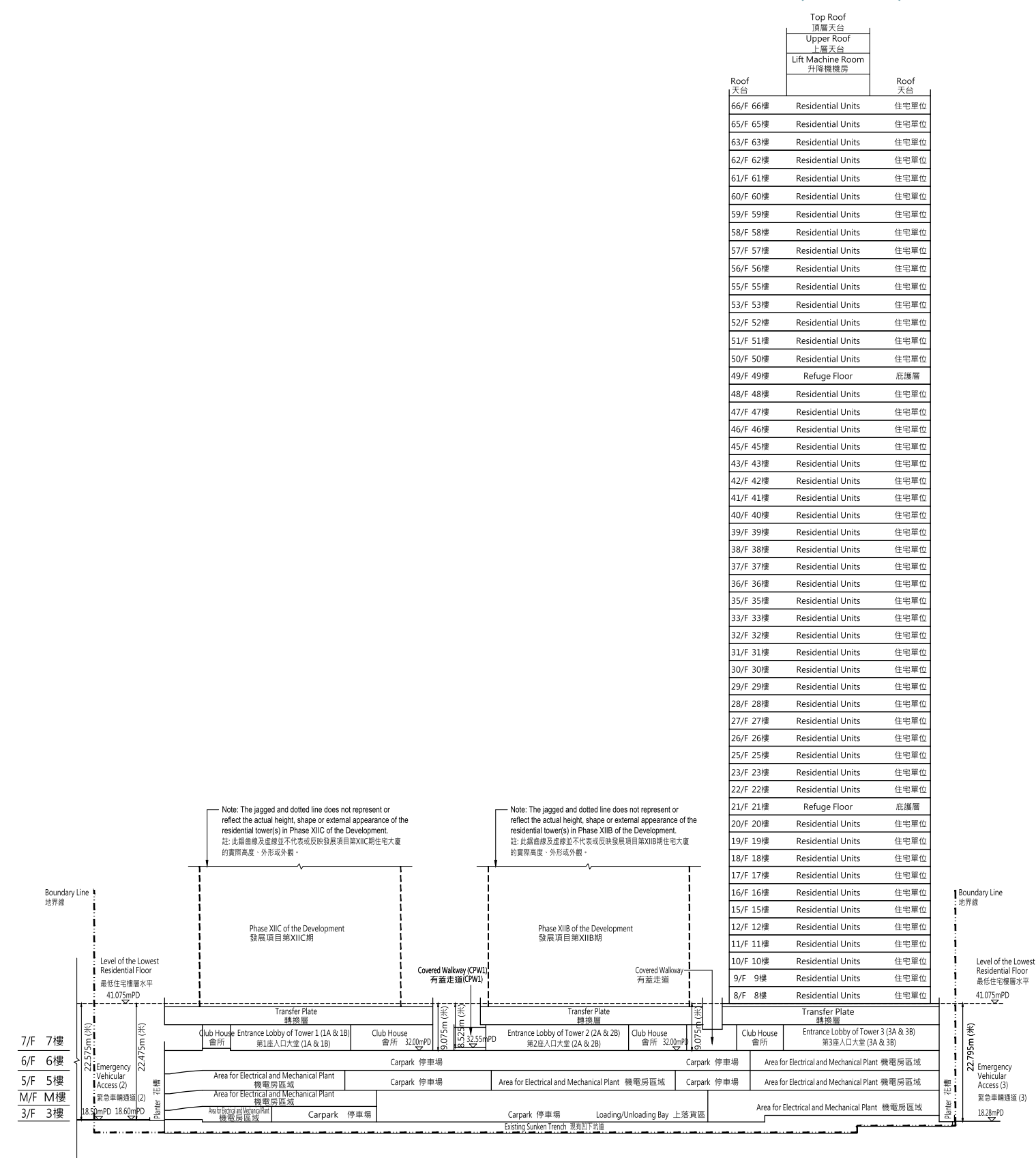
Cross-Section Plan A 橫截面圖 A
