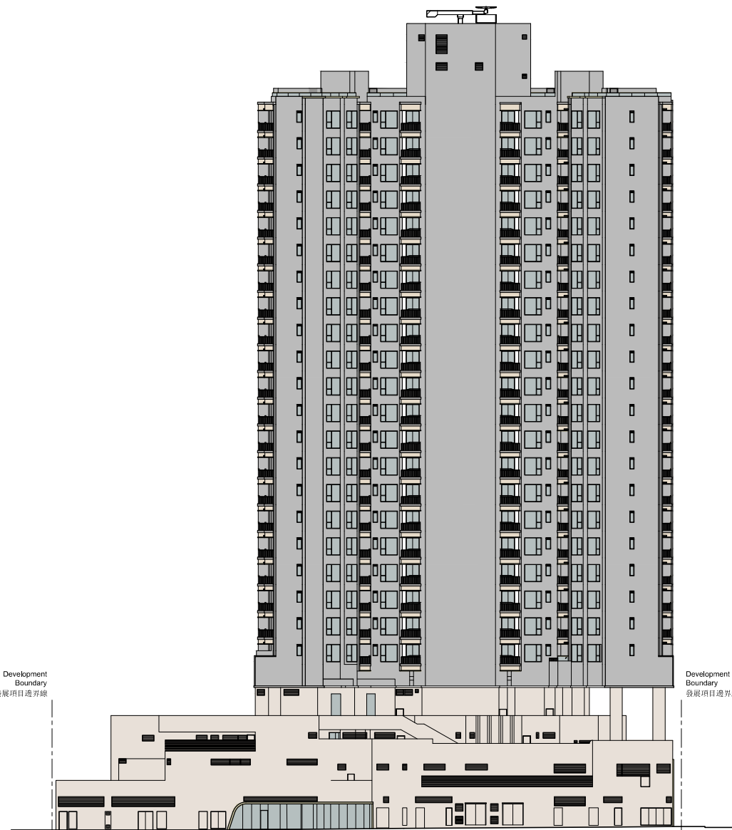
ELEVATION D 立面圖D
