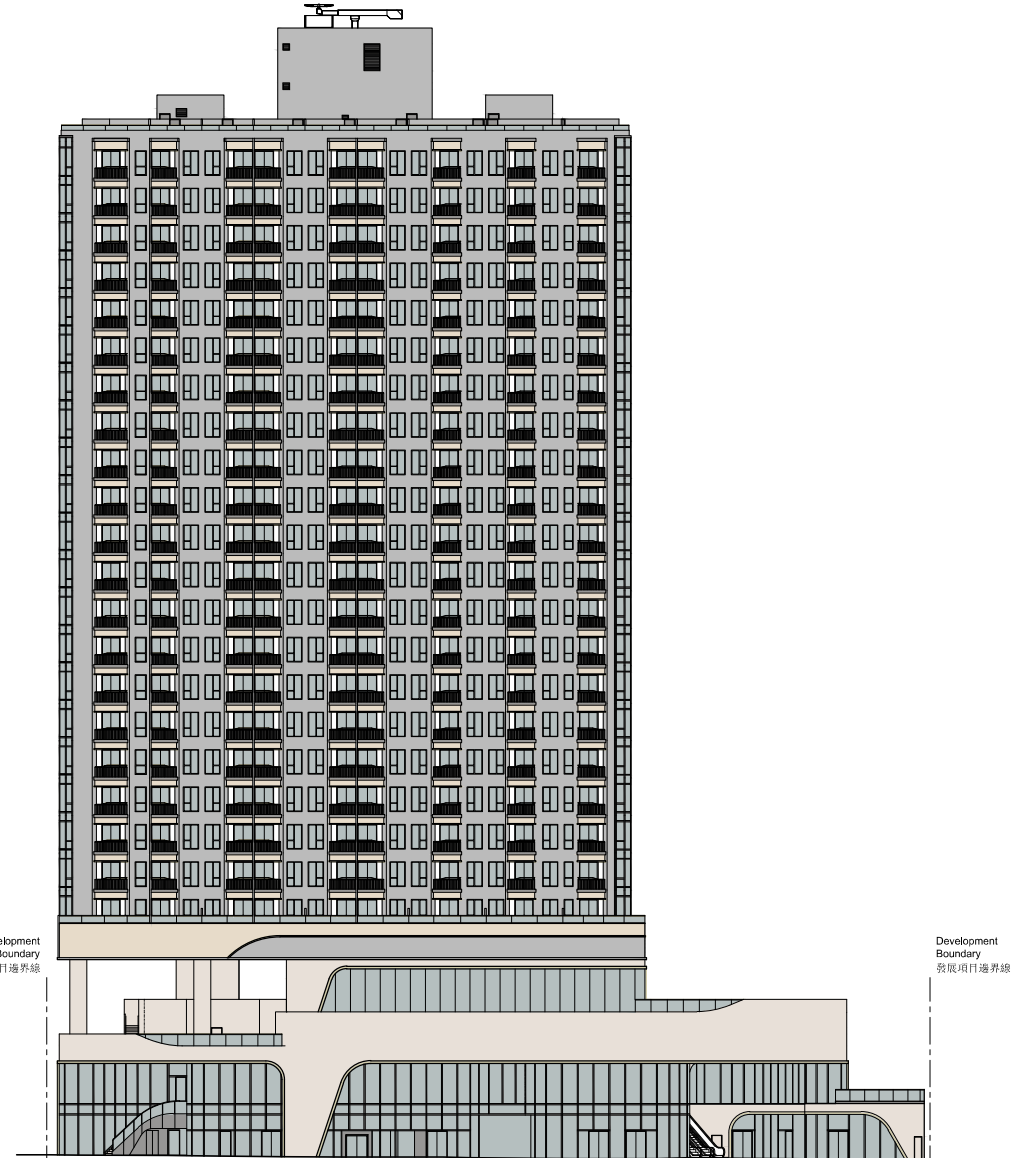
ELEVATION A 立面圖A
