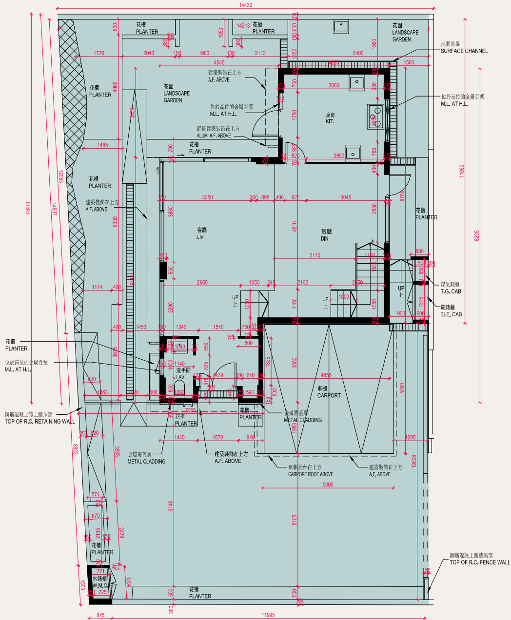
52A號洋房地下平面圖
