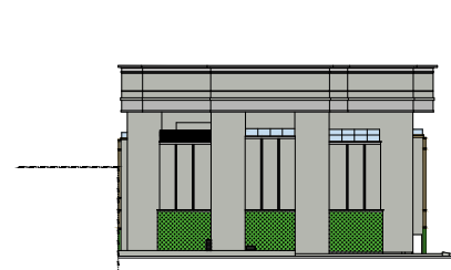
Podium Elevation E2 平台立面圖E2
