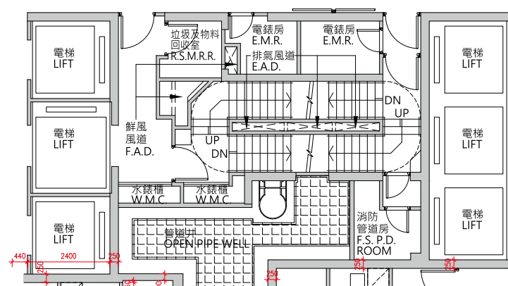
Tower 3 (3A & 3B) 66/F Part Plan 第3座(3A及3B) 66樓部分平面圖
