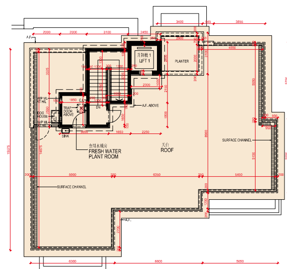
R/F AS-IS PLAN 天台現狀平面圖
