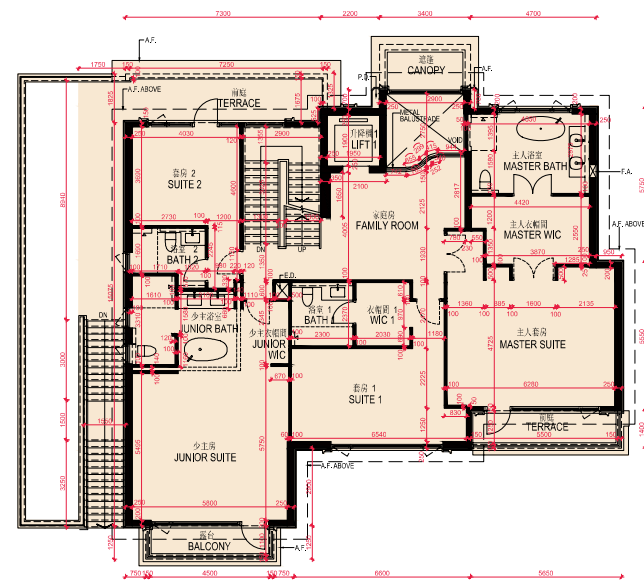
1/F FLOOR PLAN 1樓樓面平面圖
