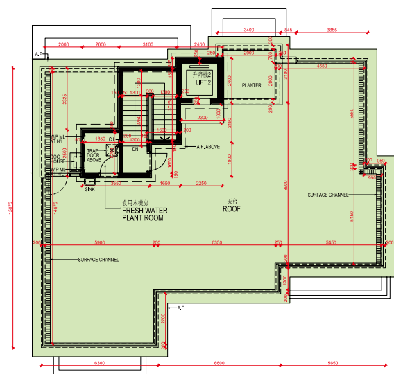
R/F AS-IS PLAN 天台現狀平面圖
