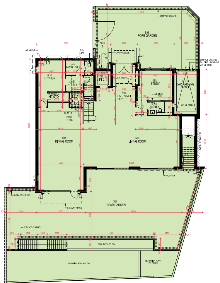
G/F FLOOR PLAN 地面層樓面平面圖
