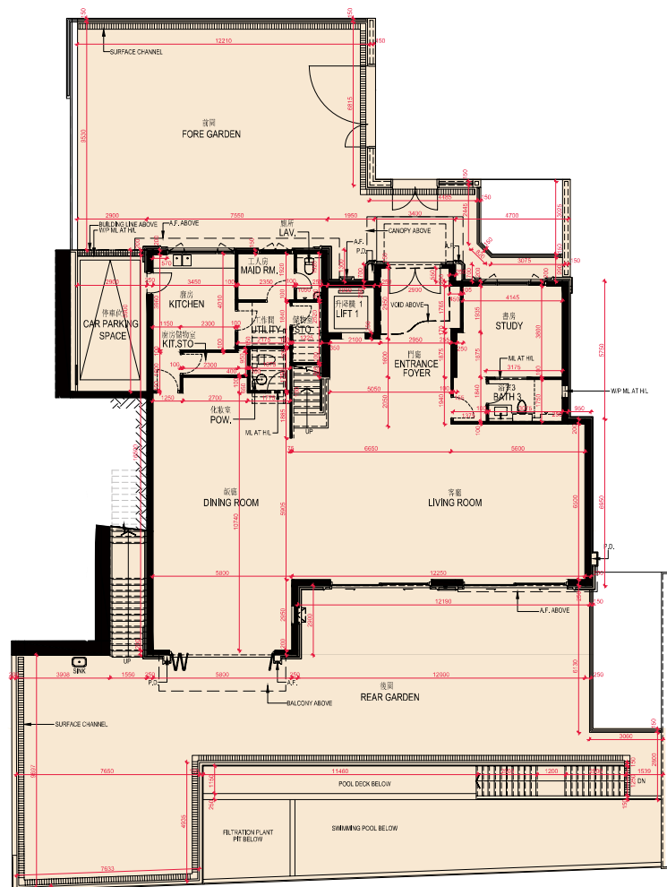
G/F FLOOR PLAN 地面層樓面平面圖
