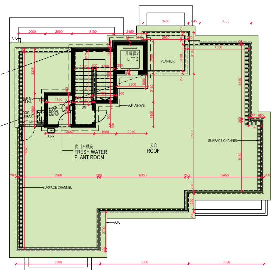
R/F FLOOR PLAN 天台樓面平面圖
