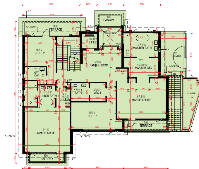
1/F AS-IS PLAN 1樓現狀平面圖
