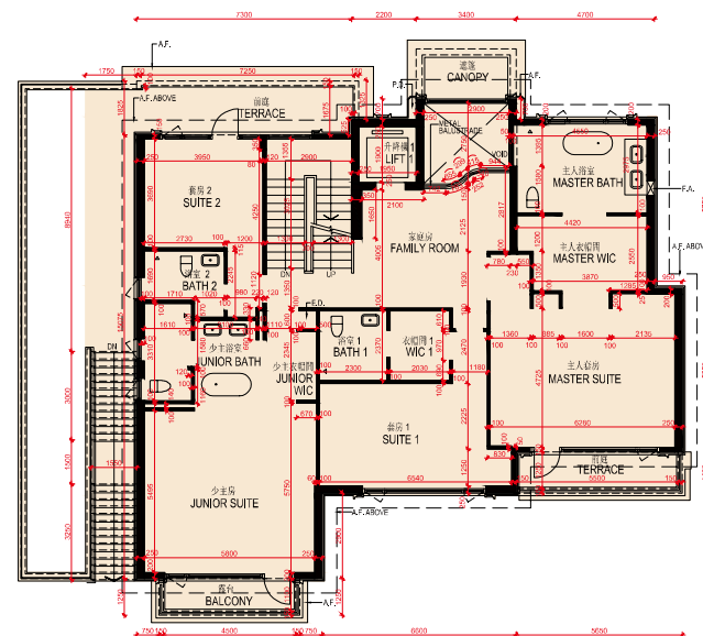
1/F AS-IS PLAN 1樓現狀平面圖
