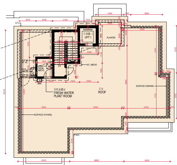
R/F FLOOR PLAN 天台樓面平面圖
