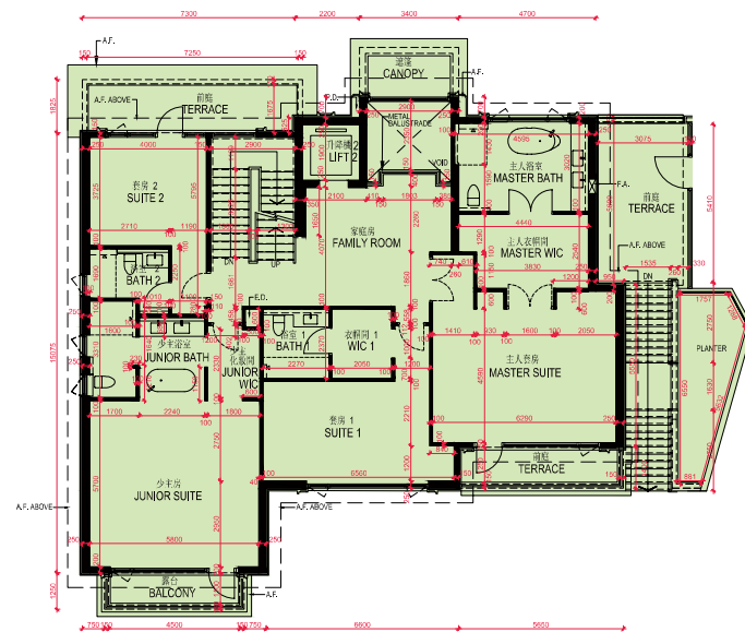
1/F FLOOR PLAN 1樓樓面平面圖
