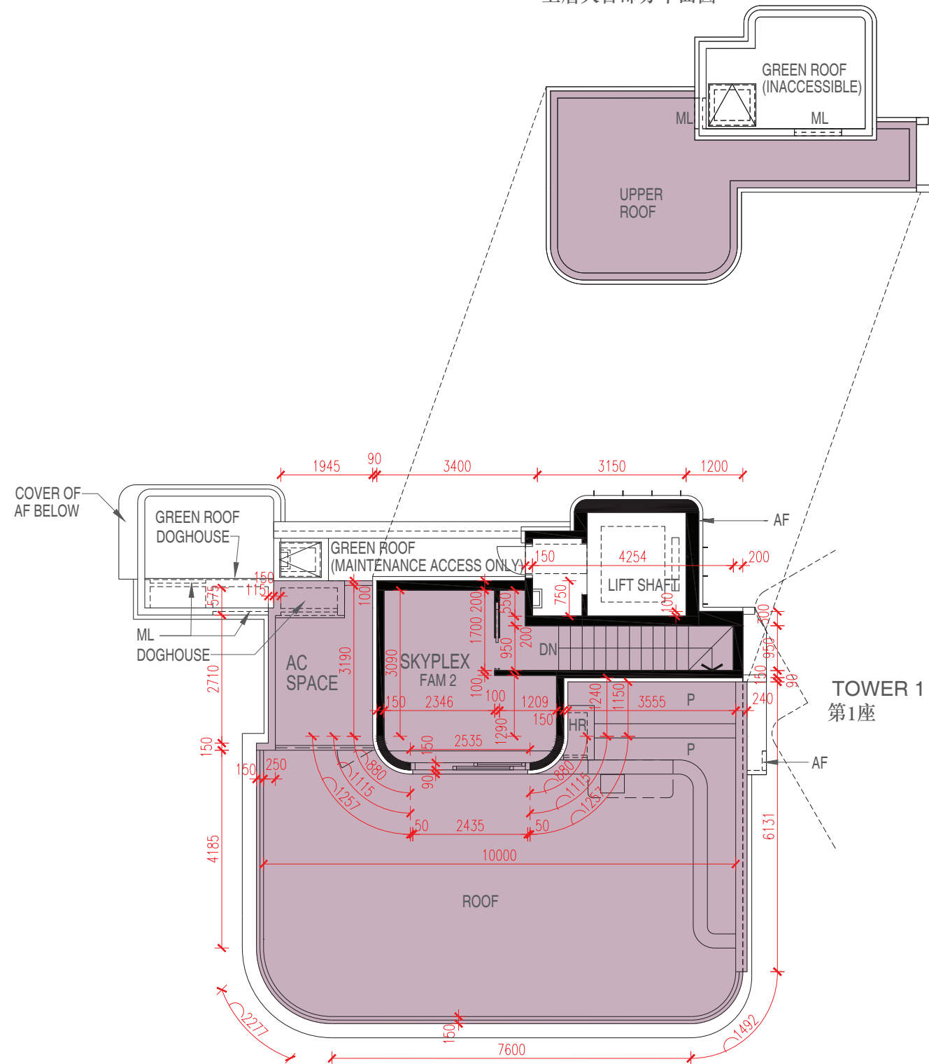
PART PLAN OF UPPER ROOF 上層天台部分平面圖
