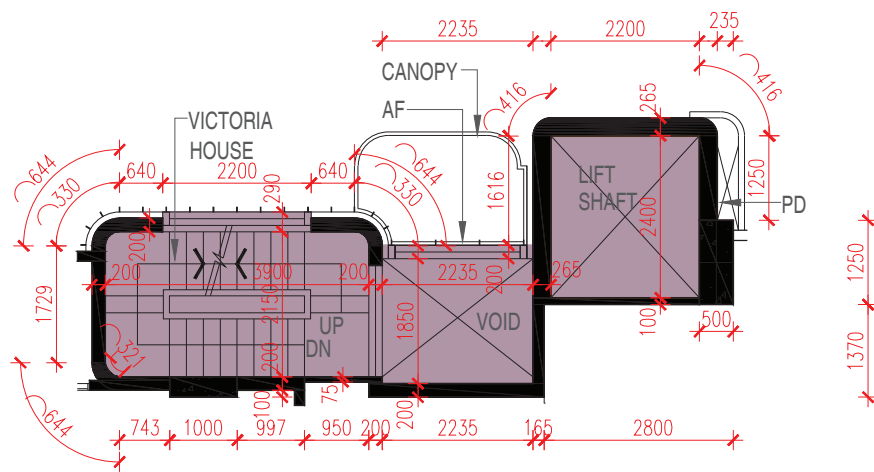
PART PLAN OF 1/F 1樓部分平面圖
