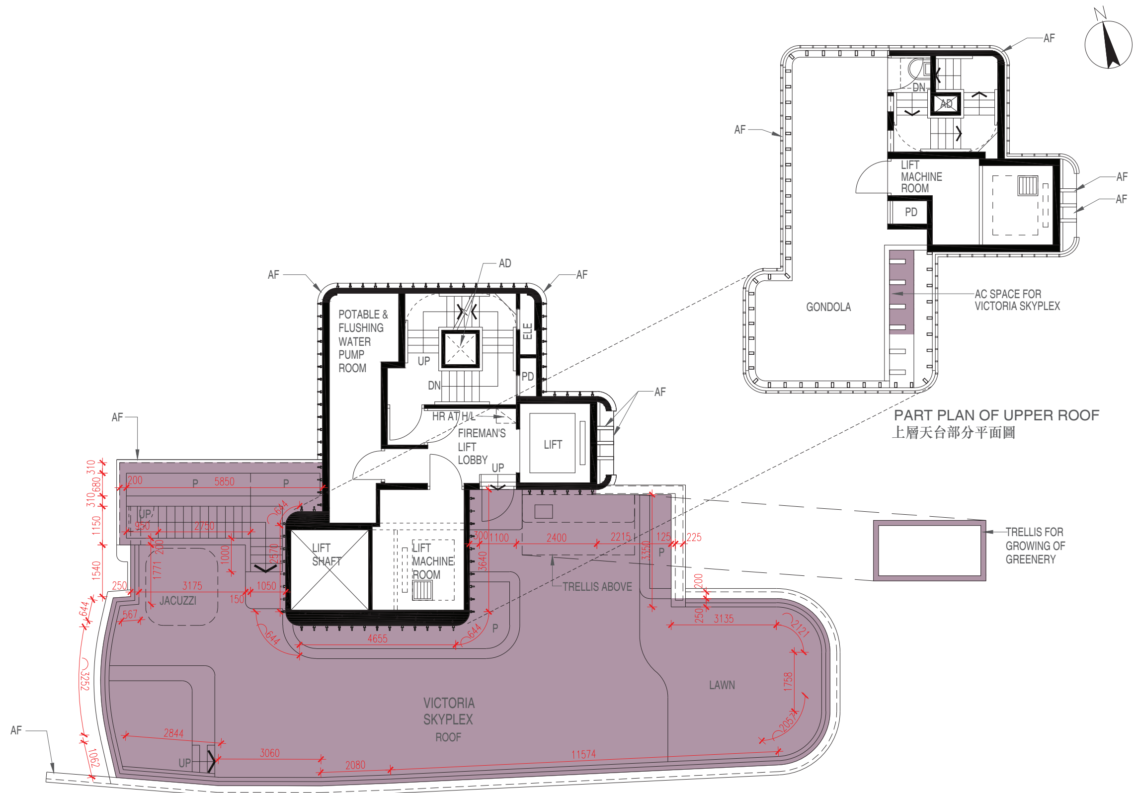
TOWER 1 ROOF 第1座 天台
