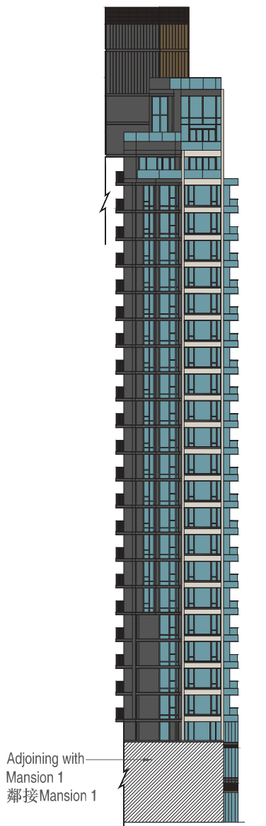
TOWER 1 ELEVATION 3 第1座 立面3
