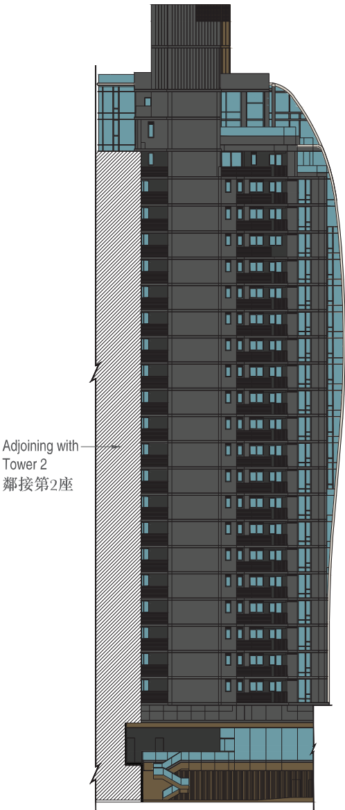
TOWER 1 ELEVATION 4 第1座 立面4
