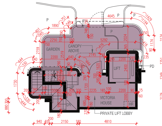
PART PLAN OF G/F 地下部分平面圖
