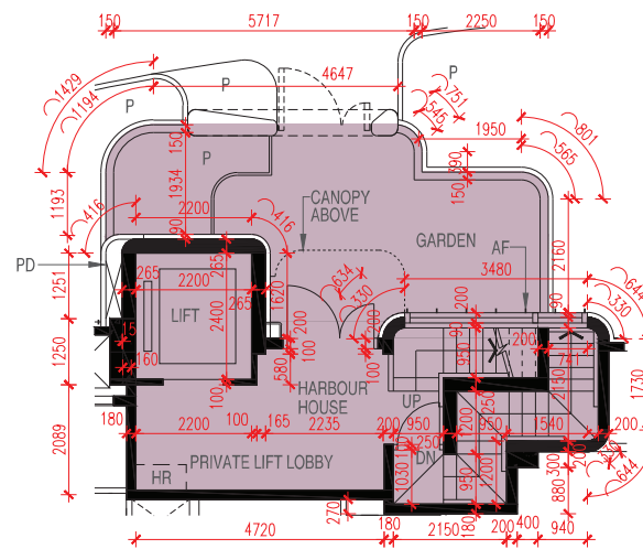
PART PLAN OF G/F 地下部分平面圖
