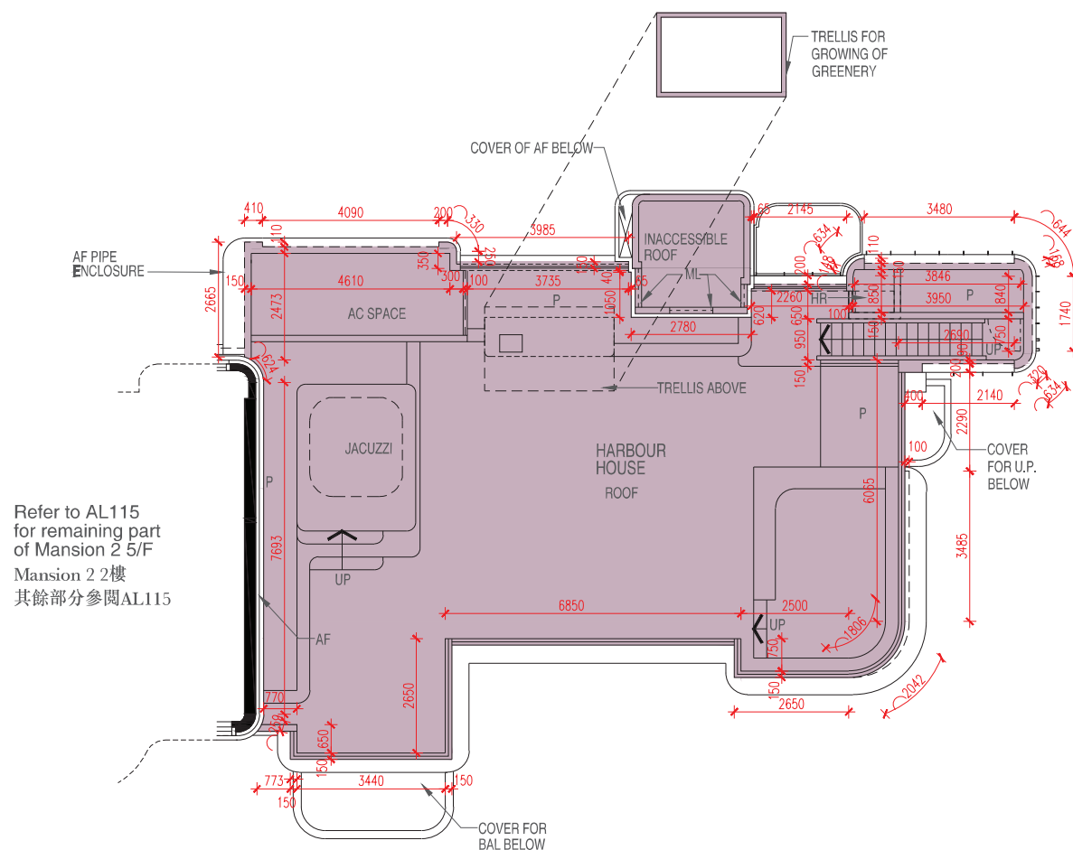
KEY PLAN FOR MANSION 2 5/F MANSION 2 5樓位置圖
