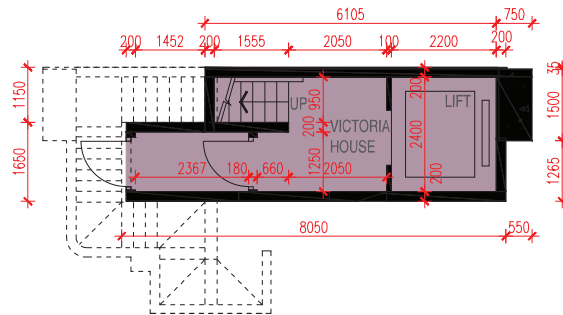
PART PLAN OF B1/F 地庫1層部分平面圖
