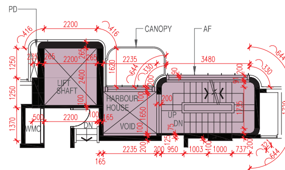
PART PLAN OF 1/F 1樓部分平面圖
