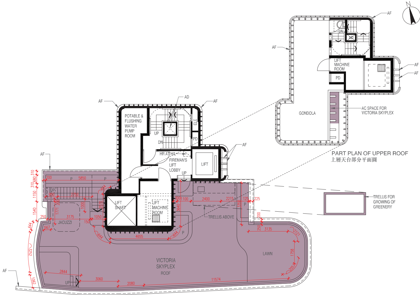
TOWER 1 ROOF 第1座 天台
