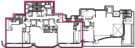
KEY PLAN FOR MANSION 2 2/F MANSION 2 2樓 位置圖
