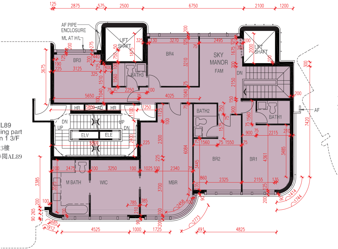
TOWER 1 第1座
