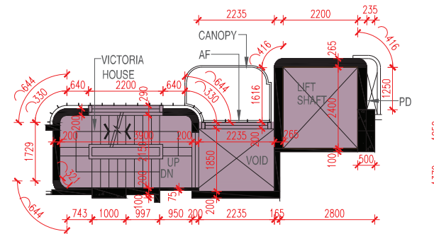
PART PLAN OF 1/F 1樓部分平面圖
