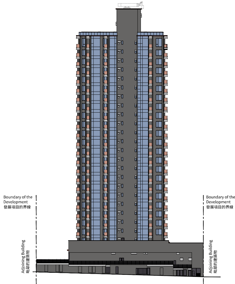
Elevation C C 立面圖
