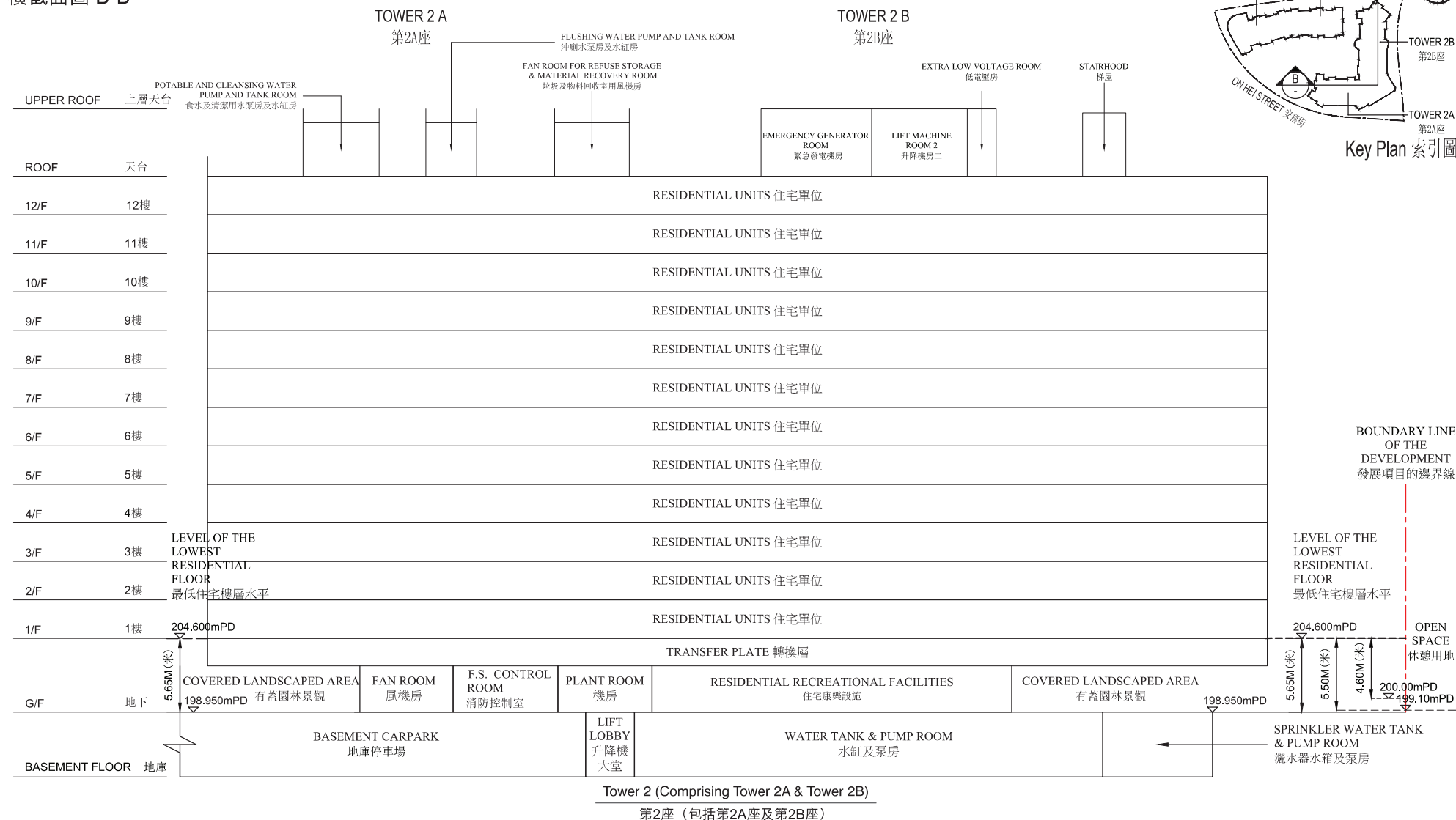
Cross Section Plan B-B 橫截面圖 B-B
