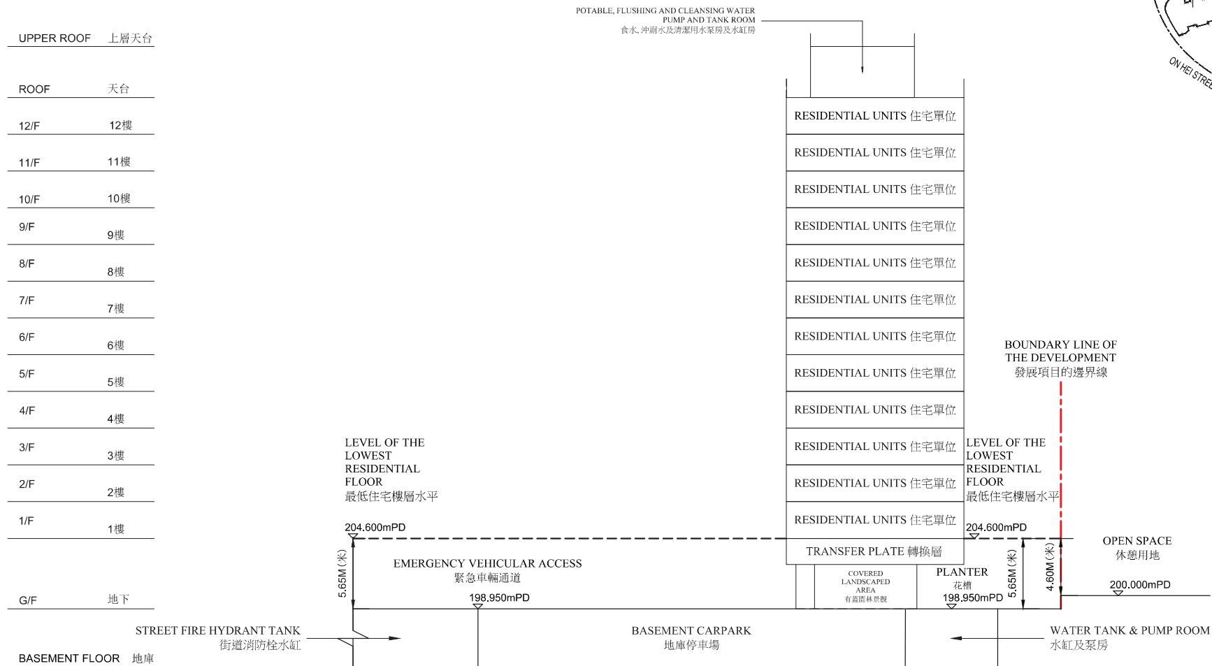
Cross Section Plan C-C 橫截面圖 C-C
