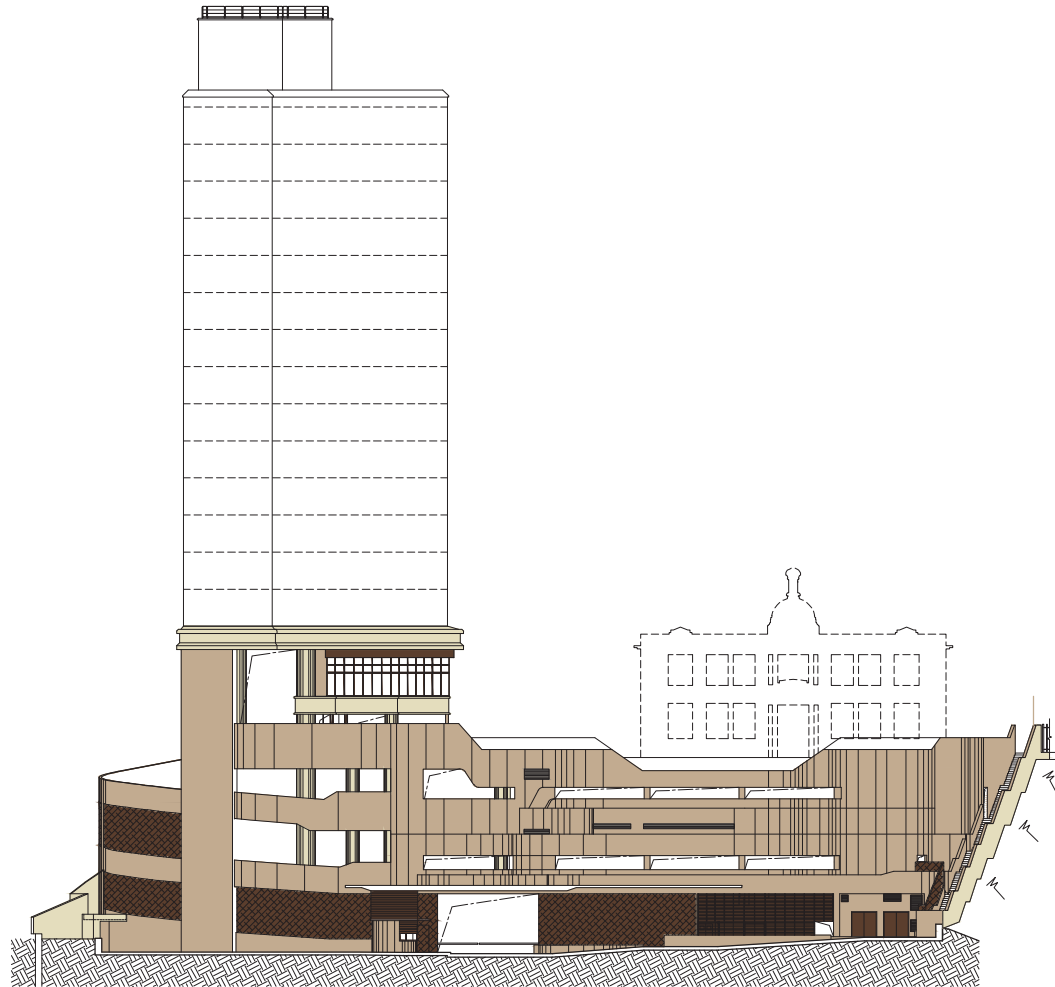
⑤ PODIUM FRONT ELEVATION 裙樓前立面
