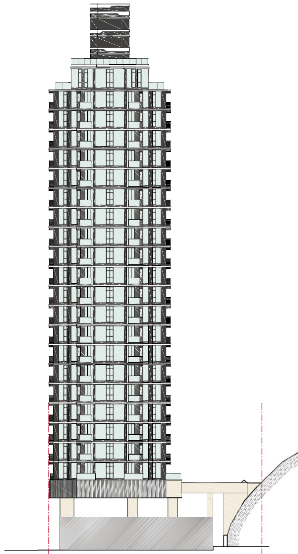
立面圖2 Elevation Plan 2
