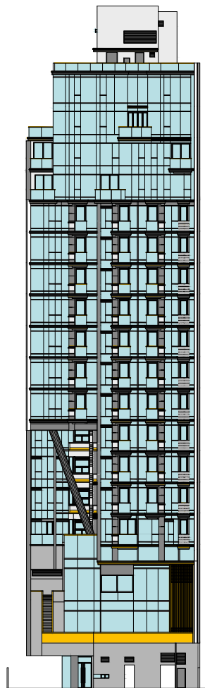
立面圖 3 ELEVATION 3
