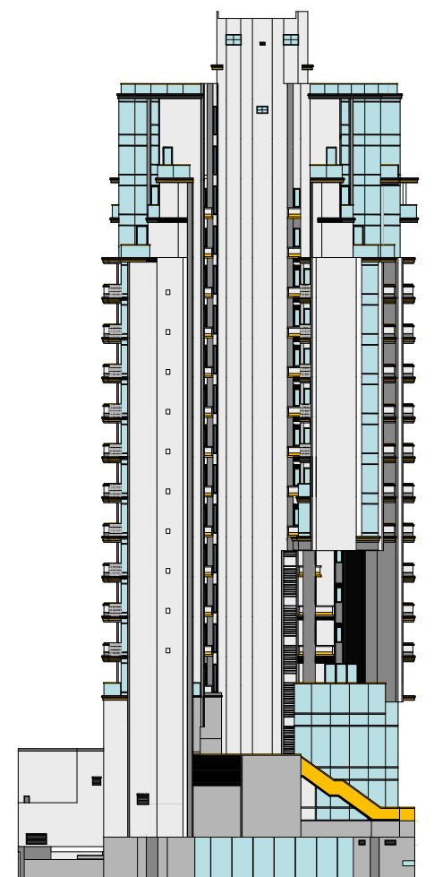
立面圖 1 ELEVATION 1
