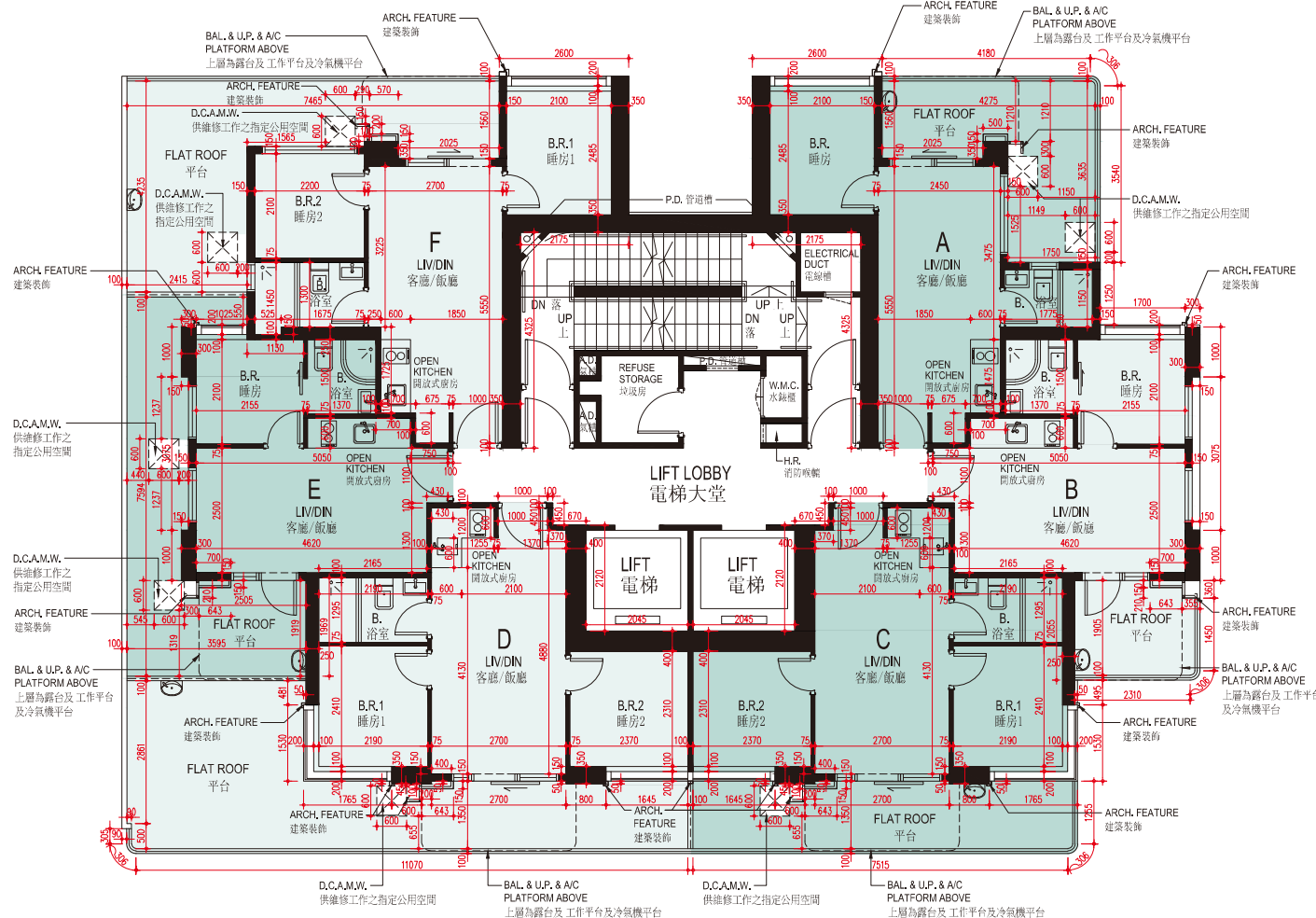
5 樓平面圖 5/F Floor Plan
