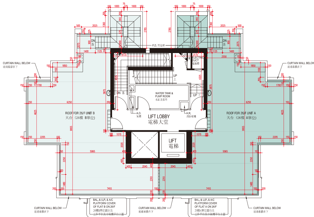
天台平面圖 Roof Floor Plan
