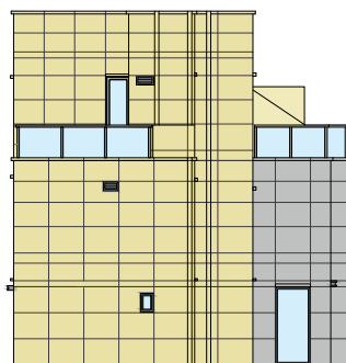
Elevation Plan 2 立面圖 2
