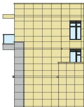
Elevation Plan 3 立面圖 3
