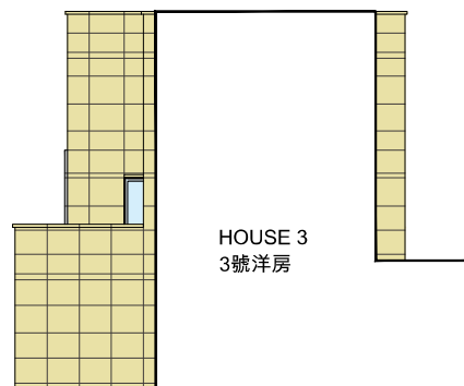
Elevation Plan 4 立面圖 4
