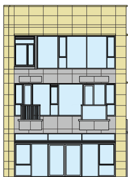
Elevation Plan 3 立面圖 3
