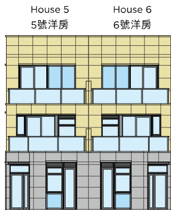
Elevation Plan 1 立面圖 1
