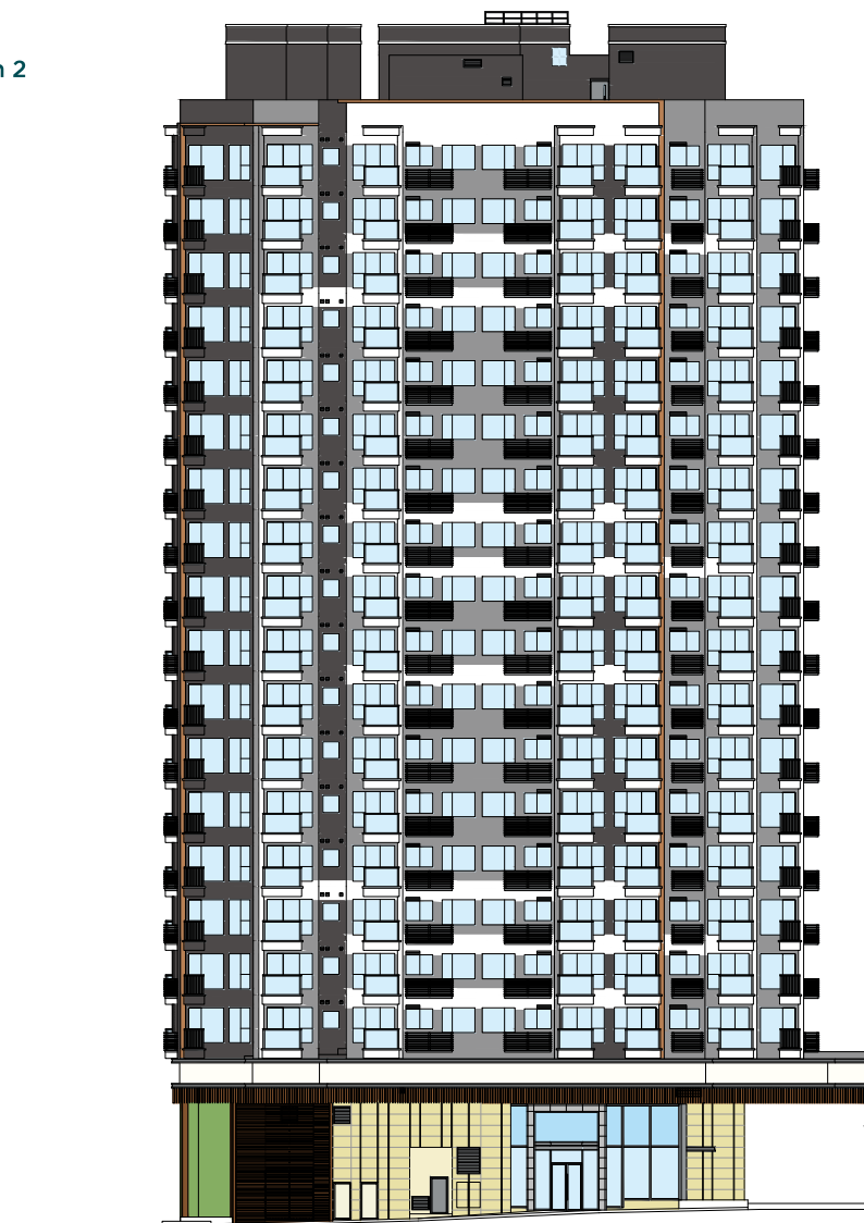
Elevation Plan Tower 1 立面圖 第1座
