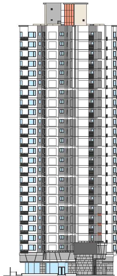
立面圖 4 ELEVATION PLAN 4
