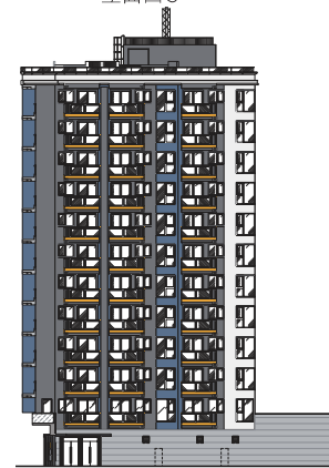
Elevation 5 立面圖5
