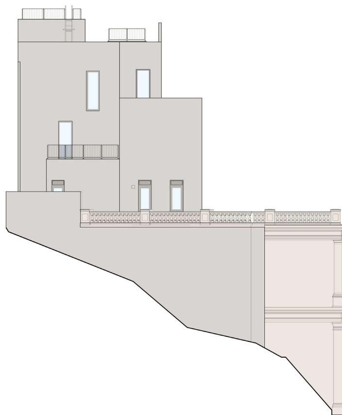
ELEVATION B 立面圖 B
