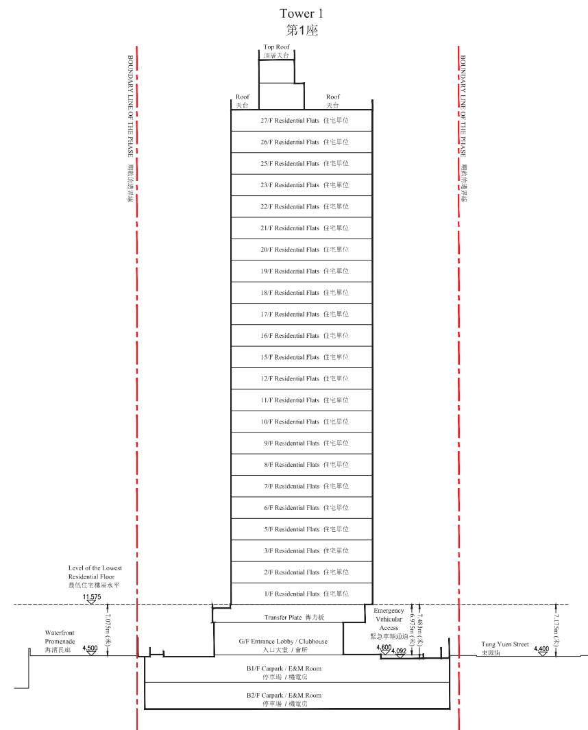
橫截面圖 B-B CROSS-SECTION PLAN B-B
