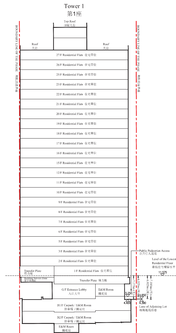
橫截面圖 A-A CROSS-SECTION PLAN A-A
