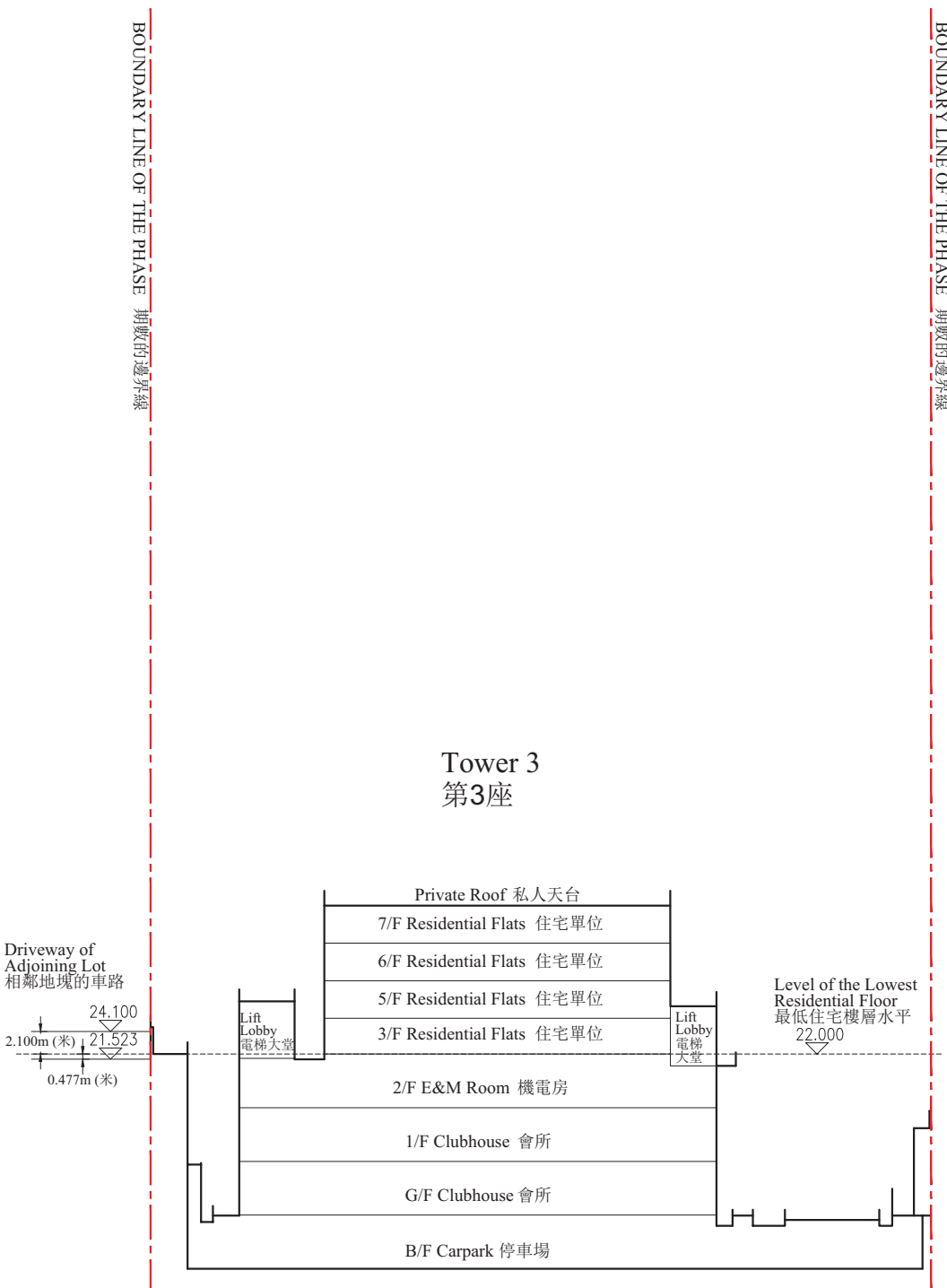
橫截面圖 D-D CROSS-SECTION PLAN D-D
