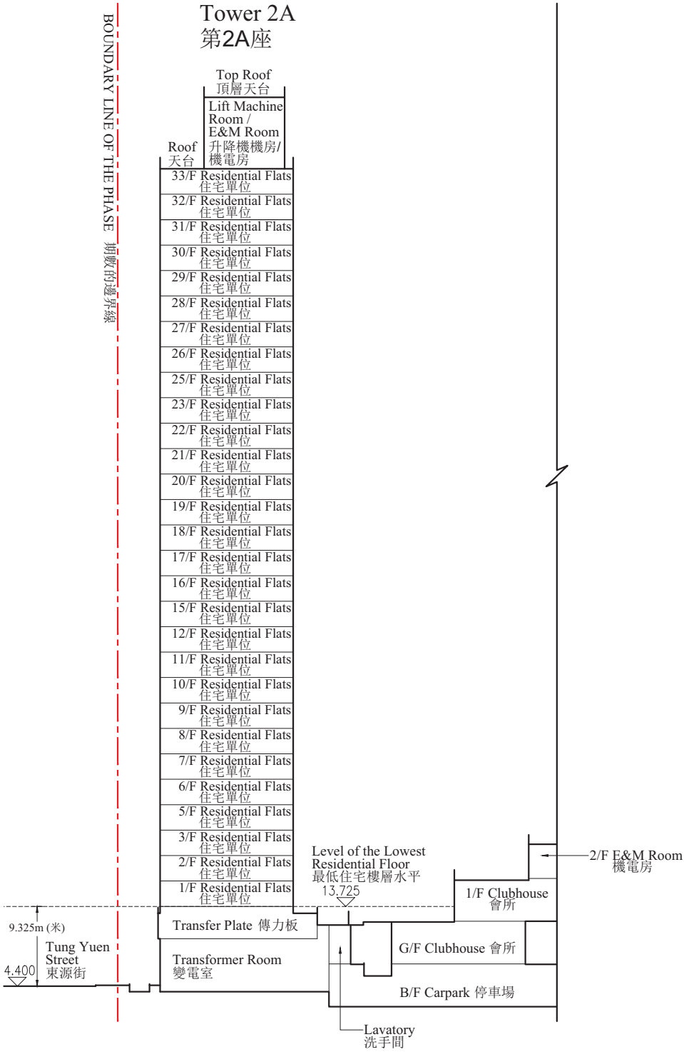
橫截面圖 B-B CROSS-SECTION PLAN B-B
