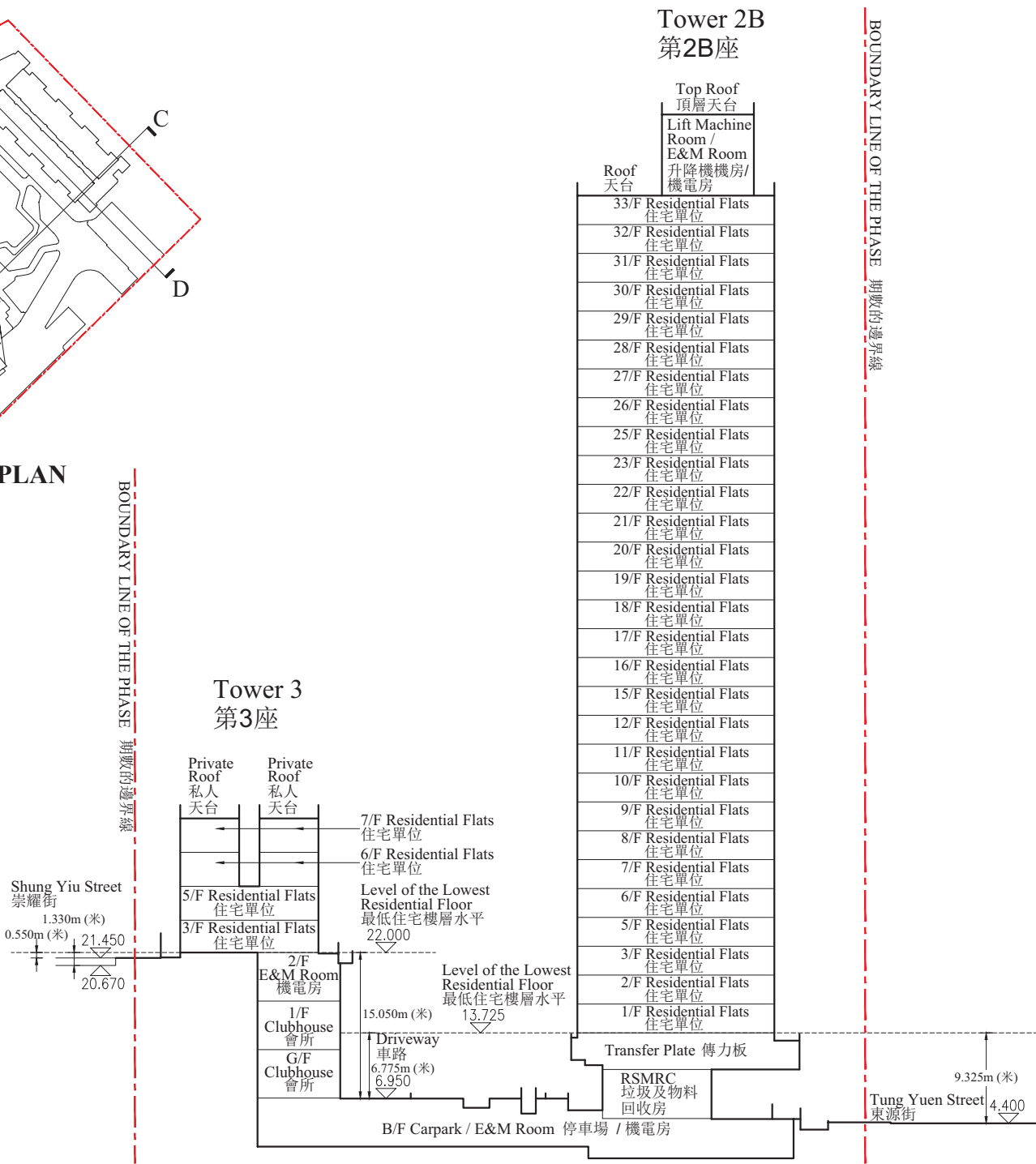
橫截面圖 C-C CROSS-SECTION PLAN C-C
