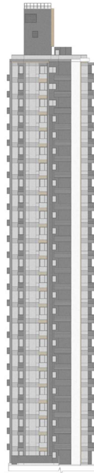
ELEVATION C 立面圖 C
