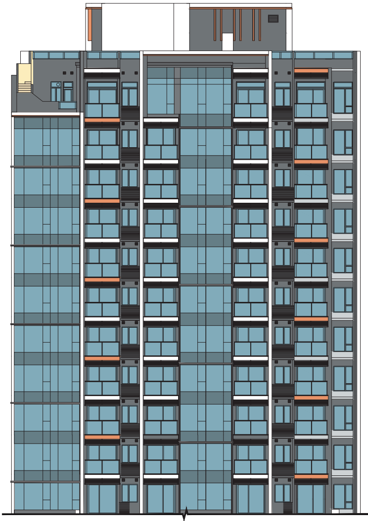
ELEVATION 4 立面 4
