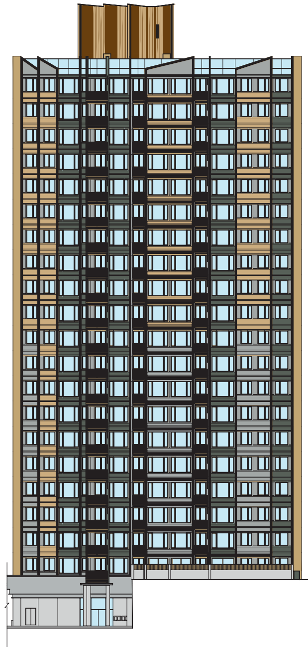
立面圖 D3 ELEVATION PLAN D3
