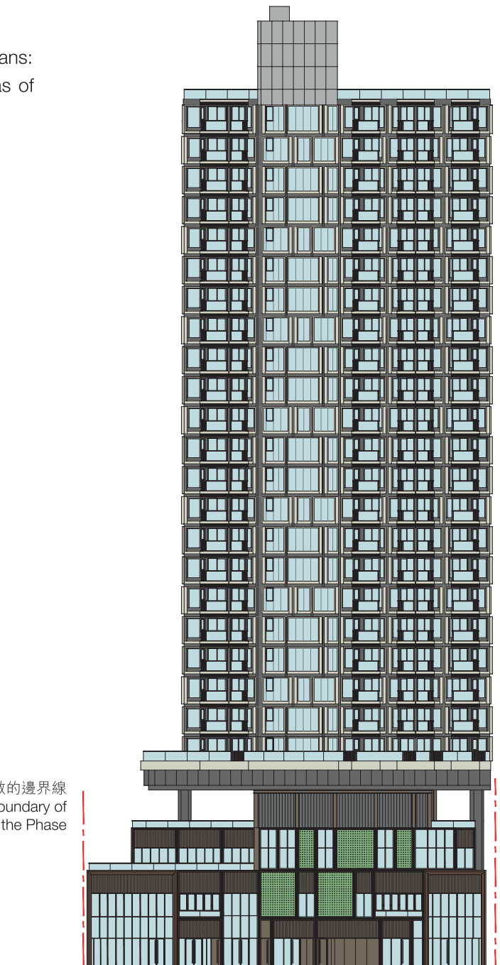
立面圖 A ELEVATION PLAN A
