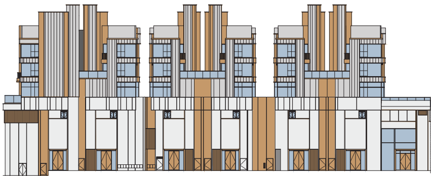
ELEVATION 3 立面圖3
