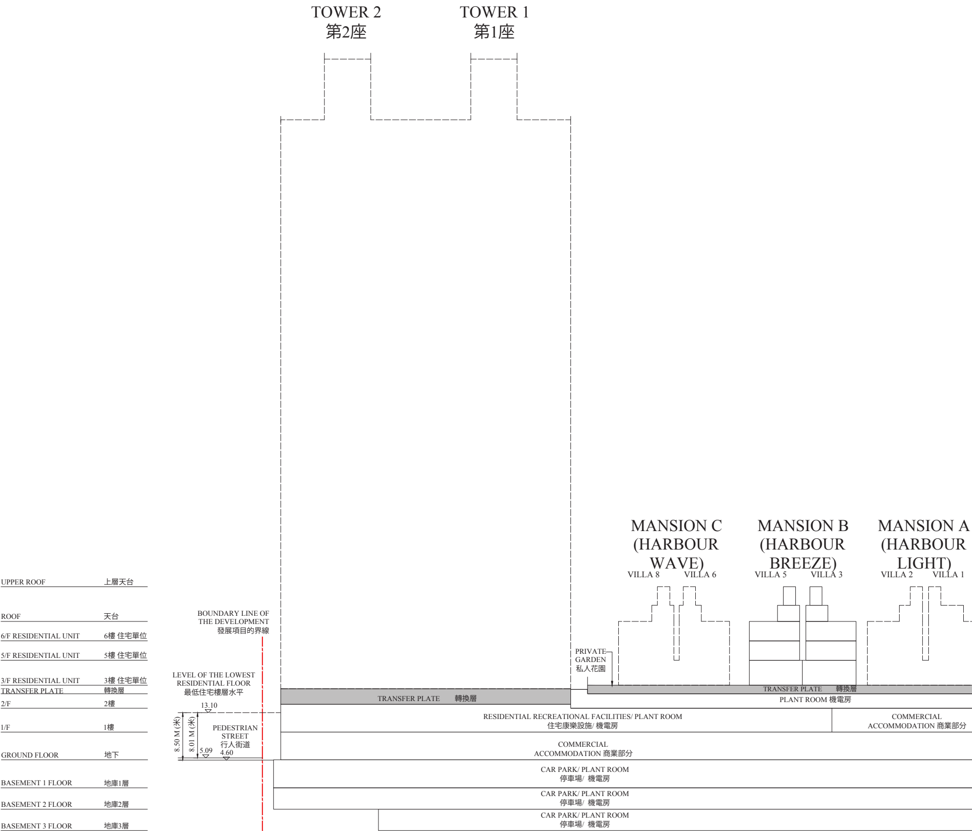
CROSS-SECTION PLAN K - K 橫截面圖 K - K
