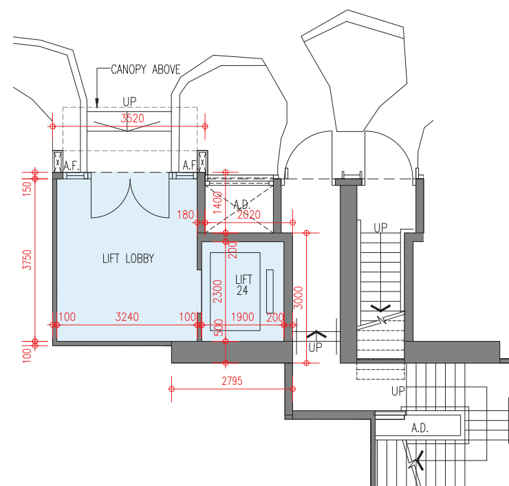
Ground Floor Plan 地下樓面平面圖
