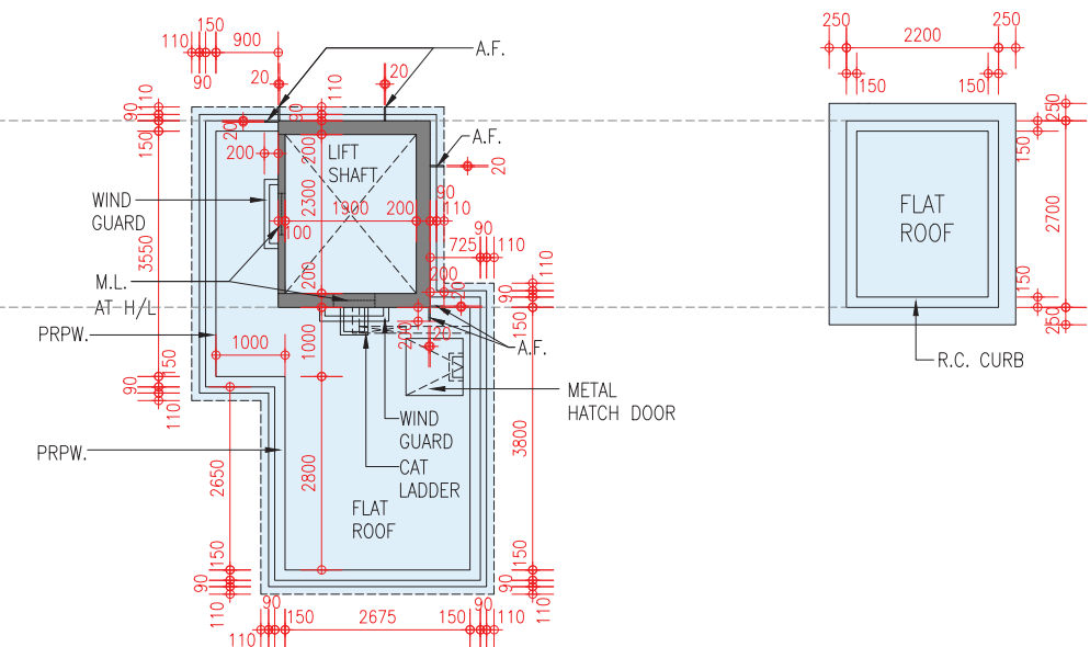
Upper Roof Floor Plan 上層天台樓面平面圖
