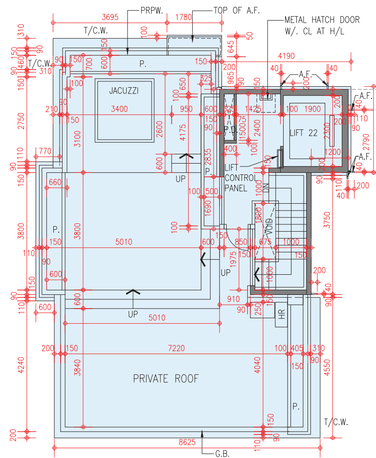
Roof Floor Plan 天台樓面平面圖
