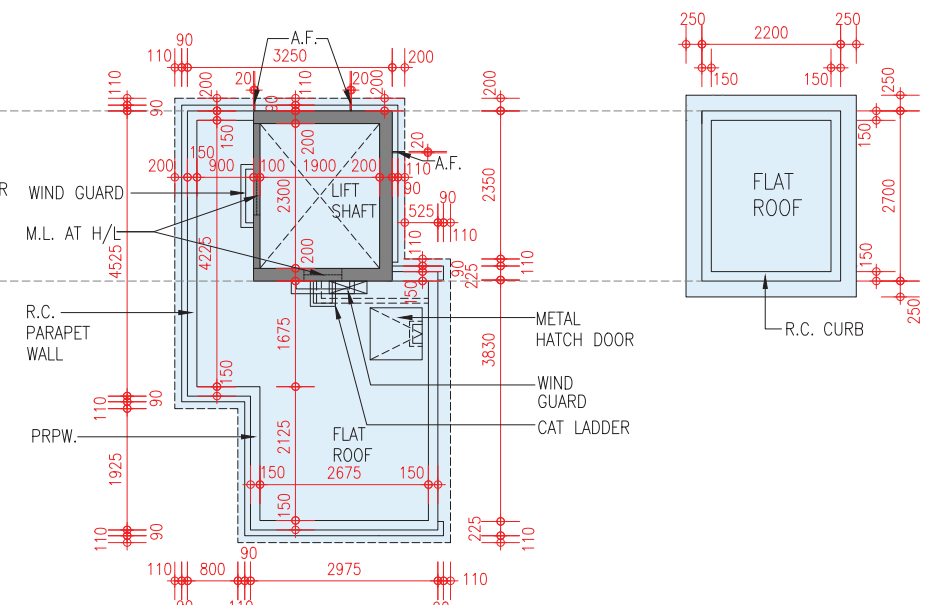
Upper Roof Floor Plan 上層天台樓面平面圖
