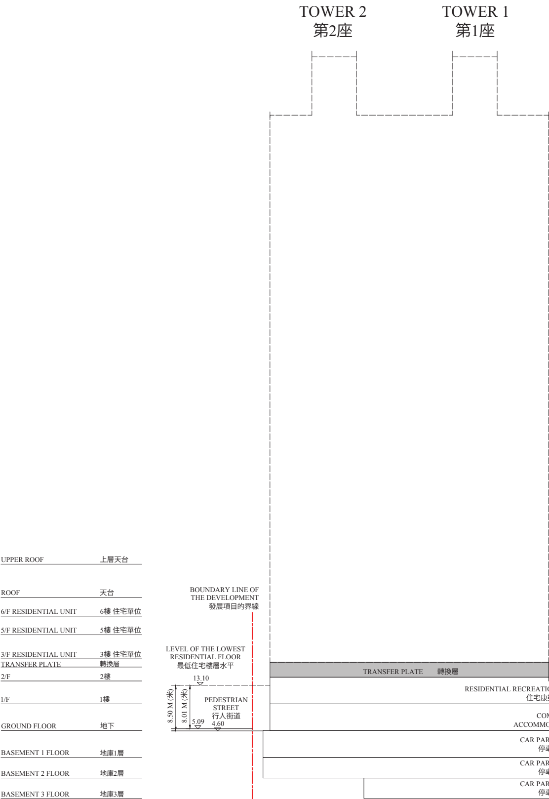
CROSS-SECTION PLAN K - K 橫截面圖 K - K
