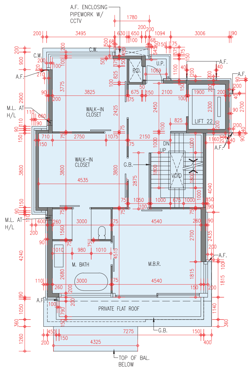
6/F Floor Plan 6樓樓面平面圖
