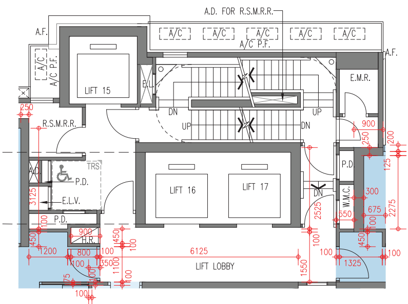
第6座37樓之部份平面圖
