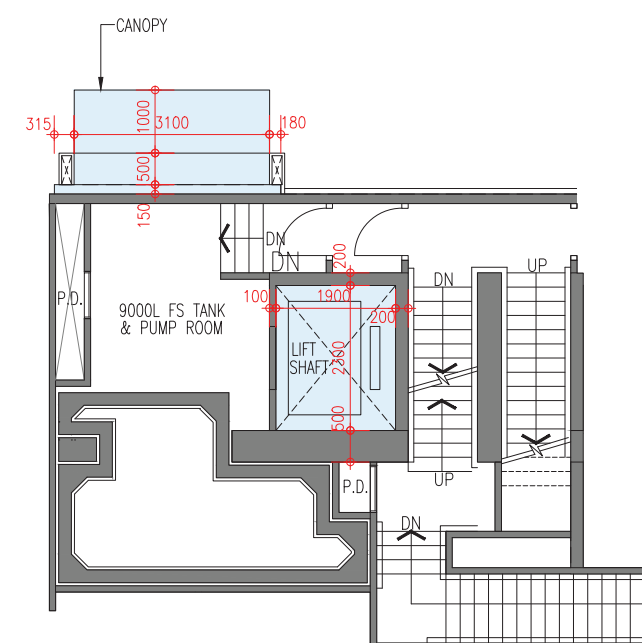
1/F Floor Plan 1樓樓面平面圖
