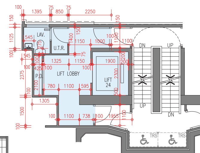
2/F Floor Plan 2樓樓面平面圖
