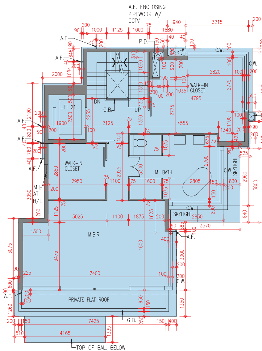
6/F Floor Plan 6樓樓面平面圖
