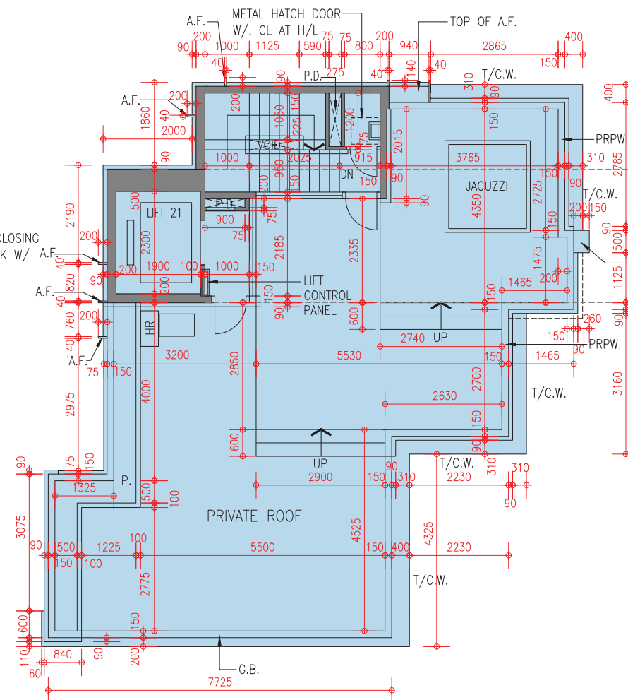
Roof Floor Plan 天台樓面平面圖
