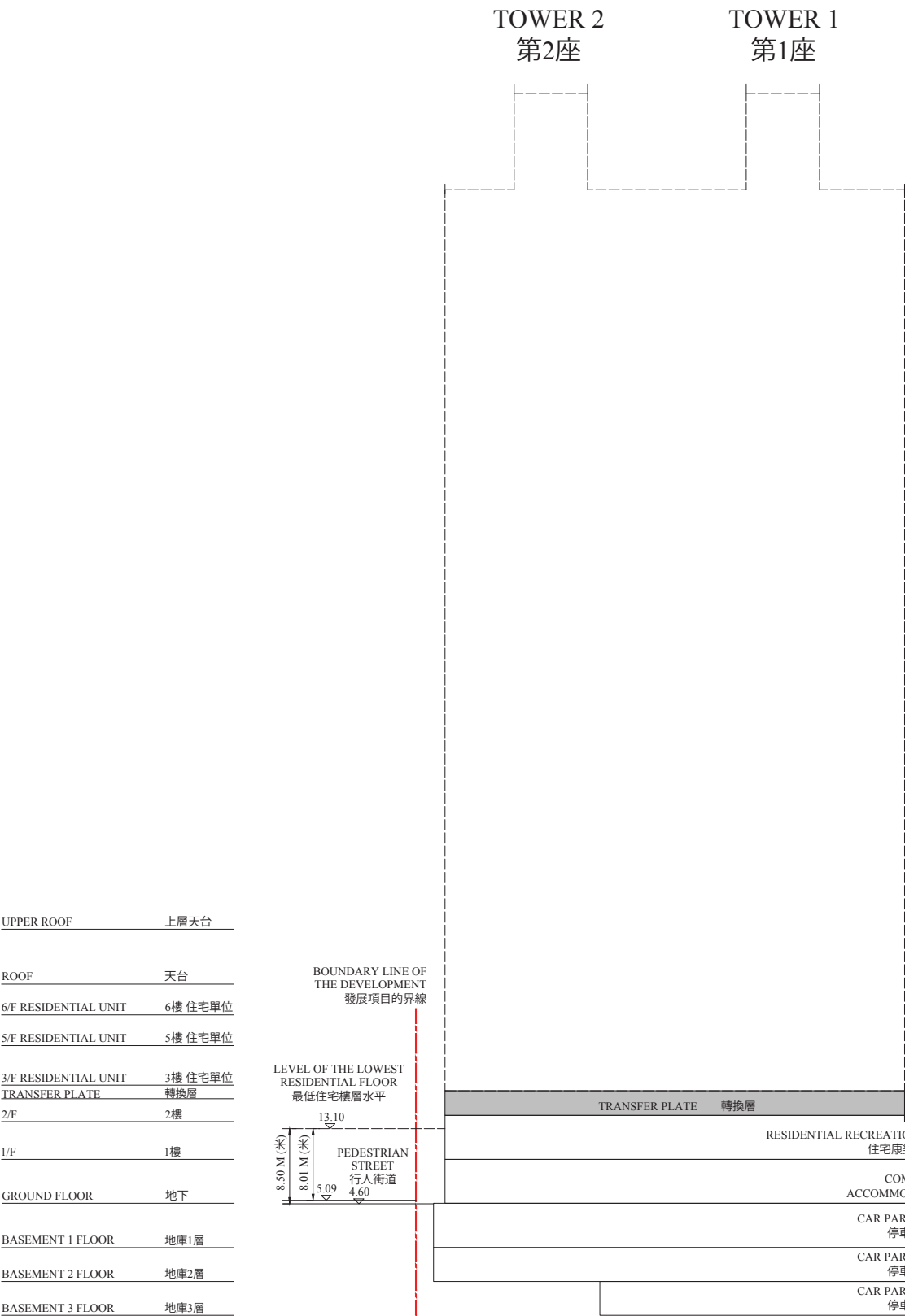
CROSS-SECTION PLAN L - L 橫截面圖 L - L
