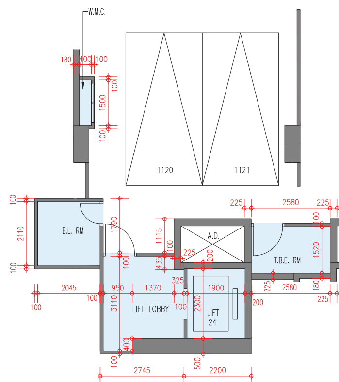
Basement 1 Floor Plan 地庫1層樓面平面圖
