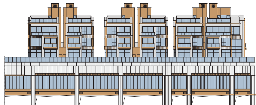
ELEVATION 1 立面圖1
