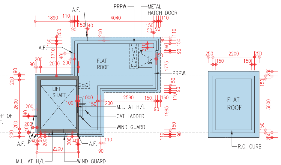
Upper Roof Floor Plan 上層天台樓面平面圖
