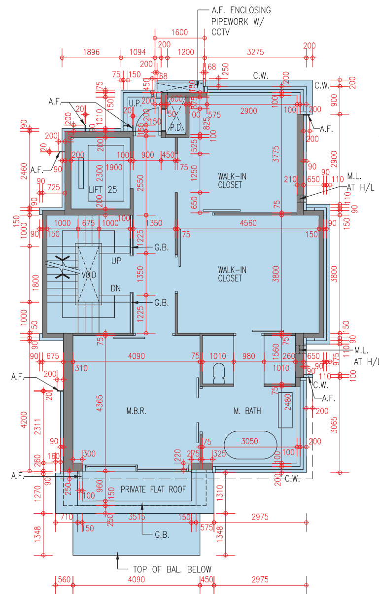
6/F Floor Plan 6樓樓面平面圖
