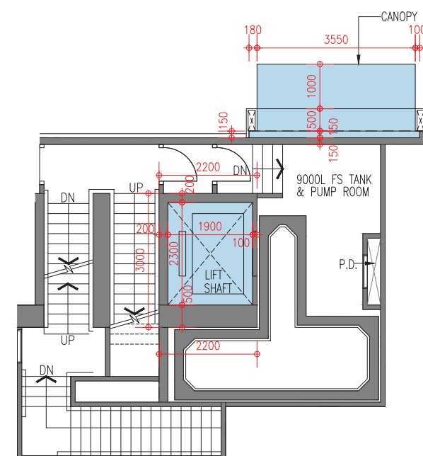
1/F Floor Plan 1樓樓面平面圖
