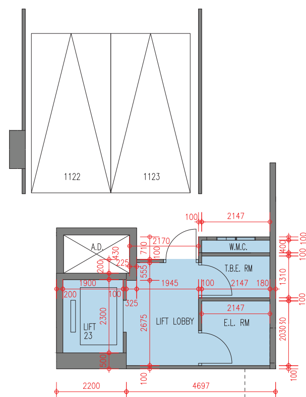
Basement 1 Floor Plan 地庫1層樓面平面圖
