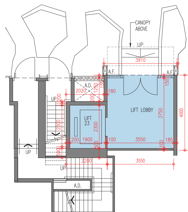
Ground Floor Plan 地下樓面平面圖
