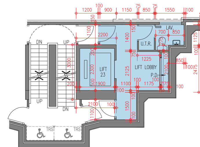
2/F Floor Plan 2樓樓面平面圖
