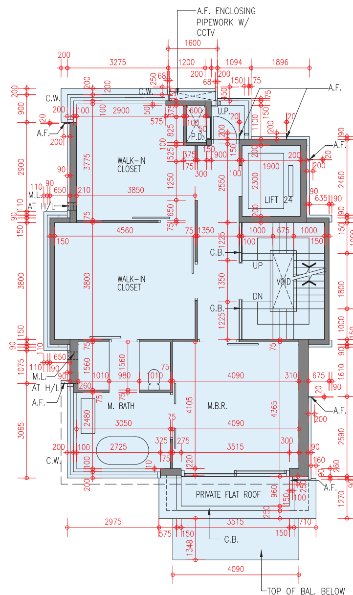
6/F Floor Plan 6樓樓面平面圖
