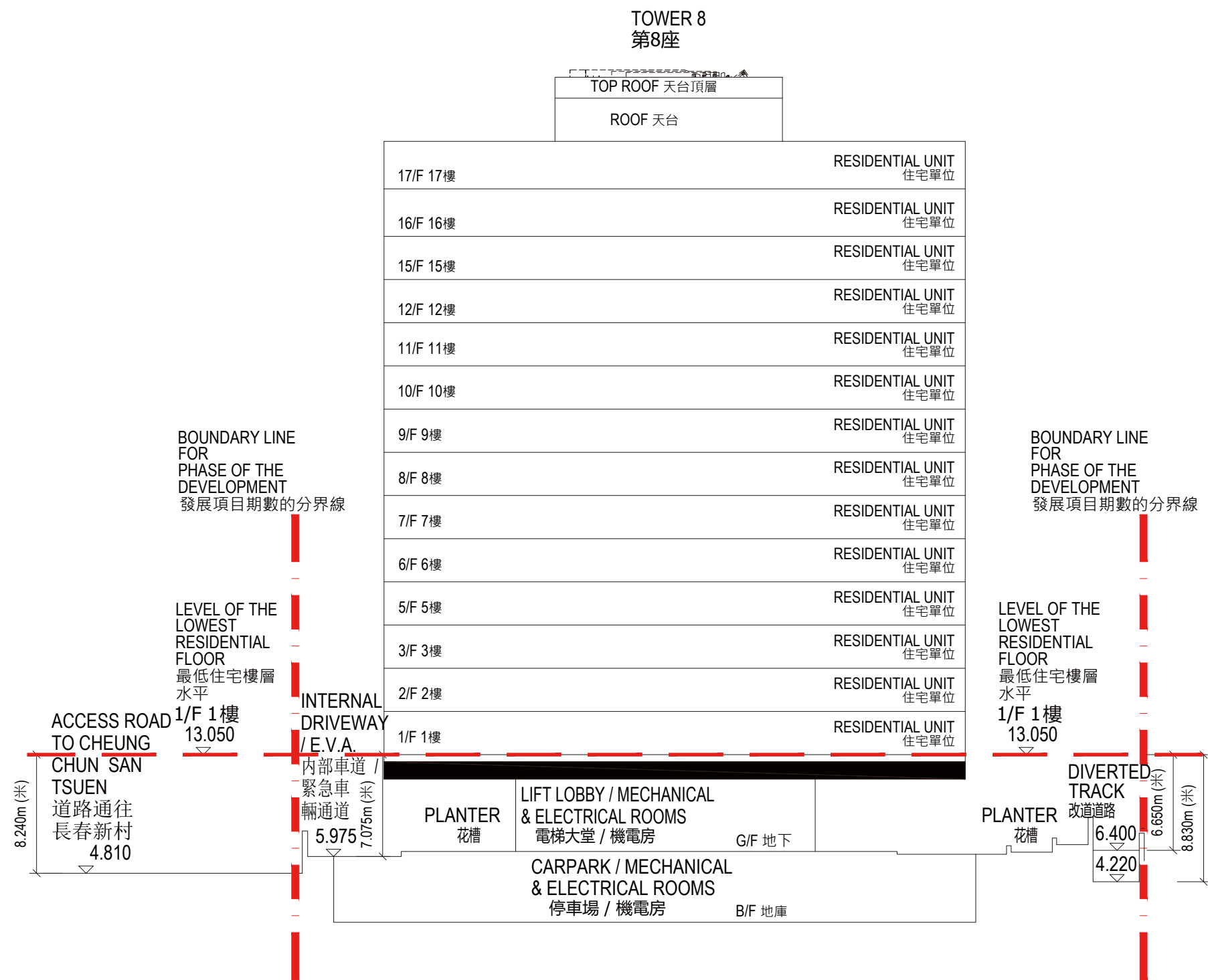
CROSS-SECTION PLAN B 橫截面圖 B
