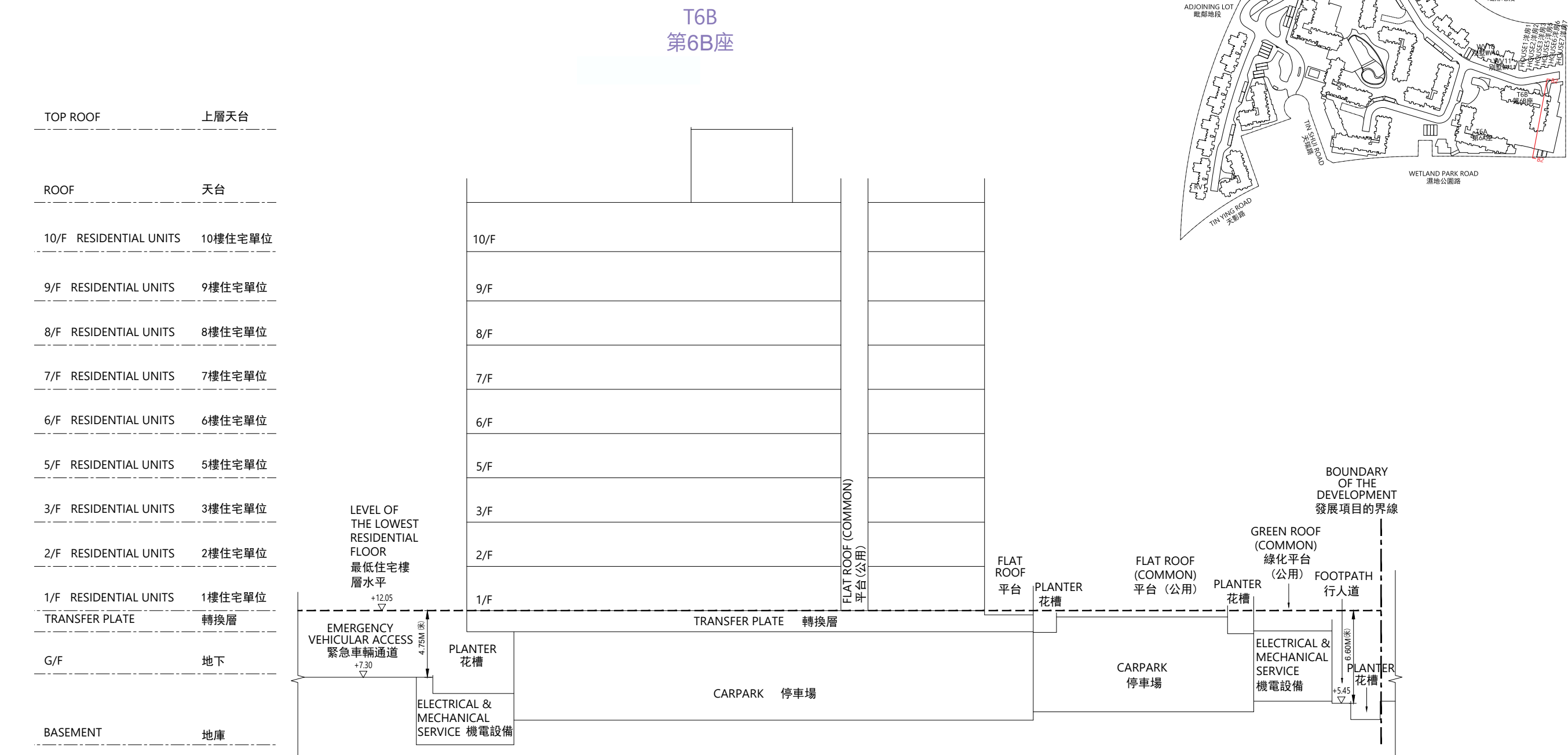
CROSS-SECTION PLAN B2 橫截面圖 B2
