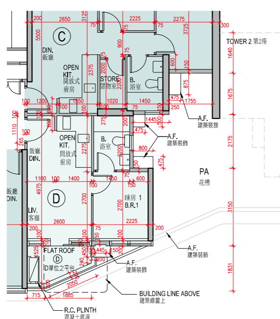
Tower 1 2/F Part Plan 第1座 2樓 局部平面圖
