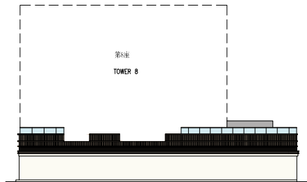
Elevation Plans 1 立面圖 1
