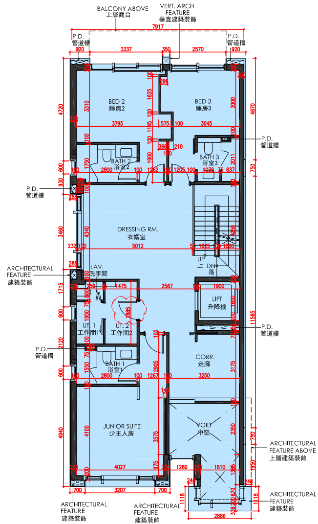
1/F AS-IS LAYOUT FLOOR PLAN 1樓現狀間隔樓面平面圖
