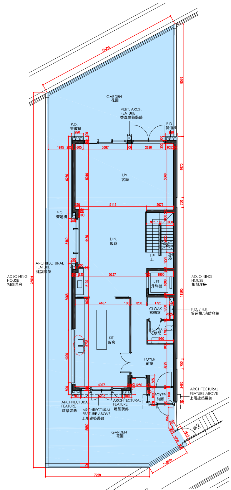
G/F AS-IS LAYOUT FLOOR PLAN 地下現狀間隔樓面平面圖
