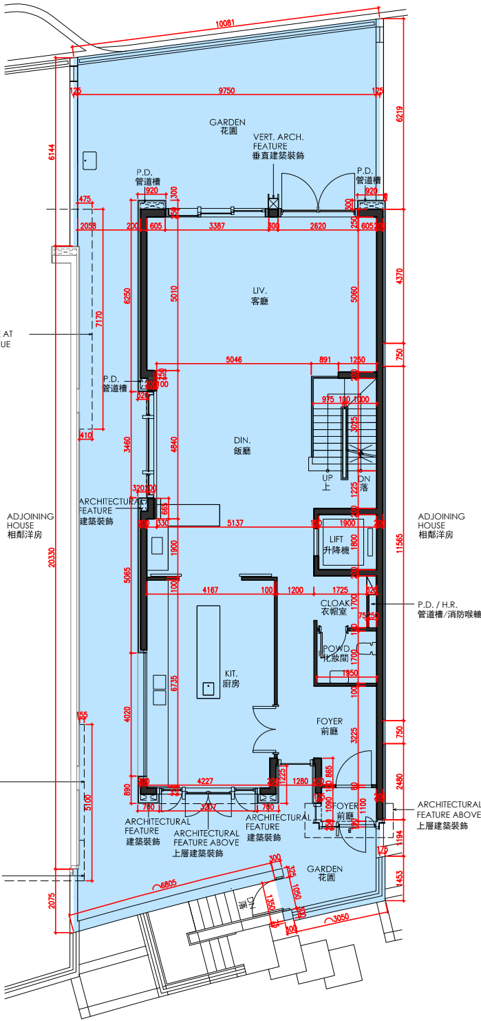
G/F FLOOR PLAN 地下樓面平面圖
